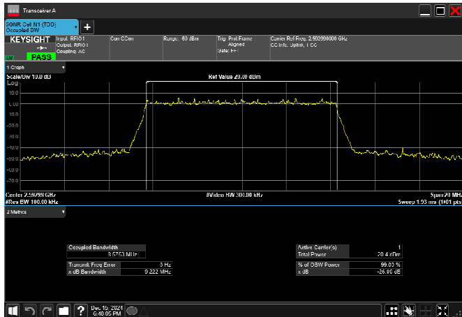
n41_10MHz_30kHz_2592.99MHz_CP-OFDM 256 QAM_RB24@0
