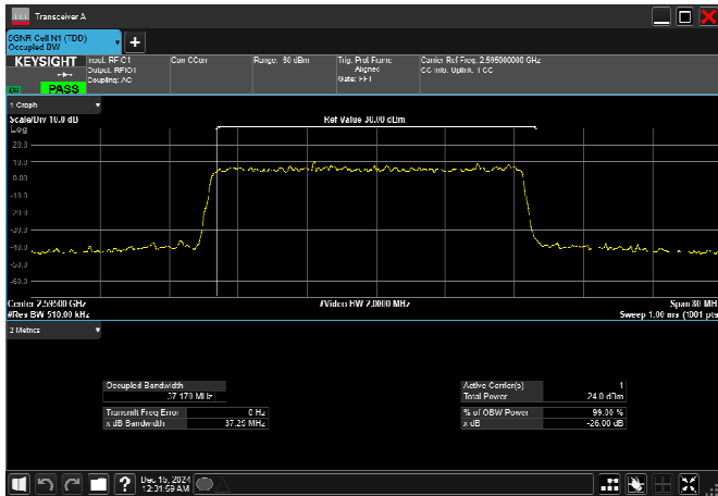
n38_40MHz_30kHz_2595MHz_CP-OFDM QPSK_RB106@0
