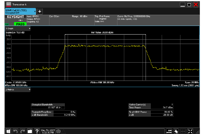
n38_10MHz_30kHz_2595MHz_DFT-s-OFDM 64 QAM_RB24@0
