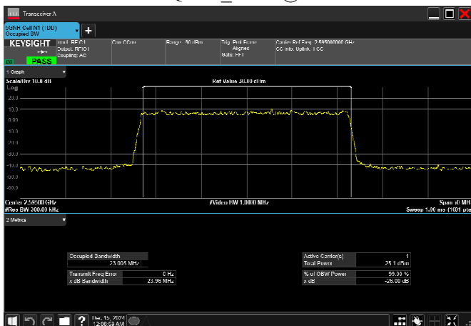
n38_25MHz_30kHz_2595MHz_DFT-s-OFDM QPSK_RB64@0
