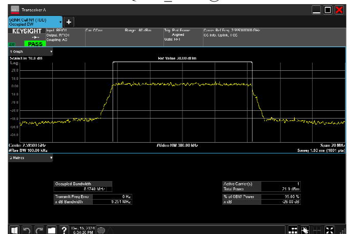
n38_10MHz_30kHz_2595MHz_CP-OFDM QPSK_RB24@0
