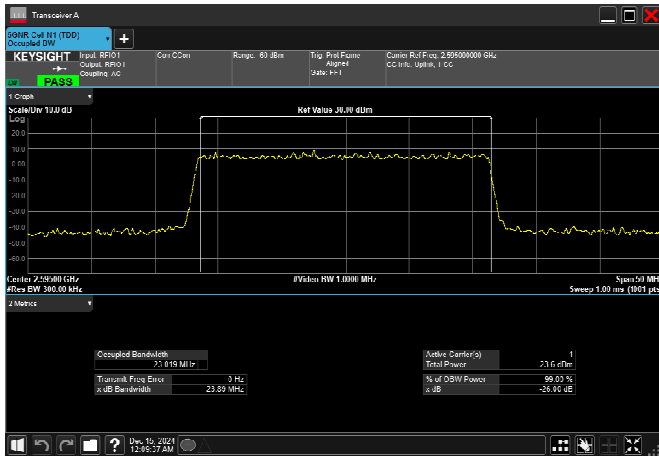
n38_25MHz_30kHz_2595MHz_CP-OFDM QPSK_RB65@0
