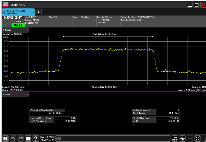
n38_20MHz_30kHz_2595MHz_CP-OFDM 256 QAM_RB51@0
