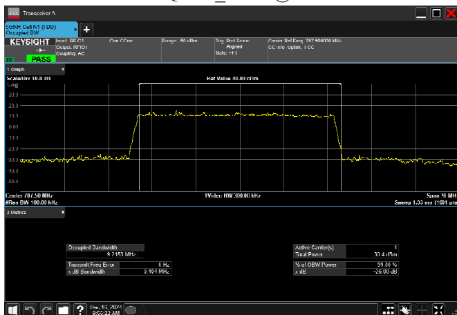
n12_10MHz_15kHz_707.5MHz_DFT-s-OFDM QPSK_RB50@0
