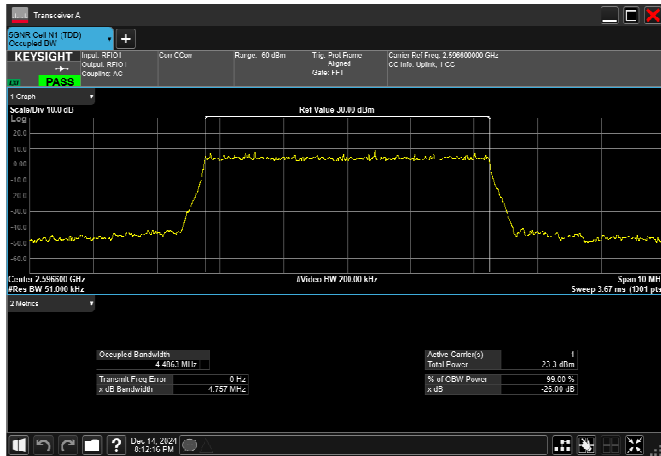
n38_5MHz_15kHz_2595MHz_CP-OFDM QPSK_RB25@0
