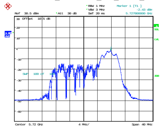
802.11ax20_5720MHz_RU_52/40_Chain 1
