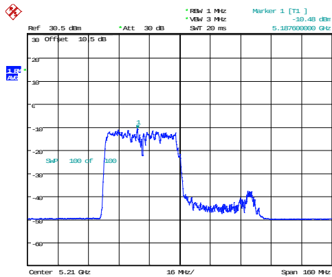
802.11ax80_5210MHz_RU_484/65_Chain 0
