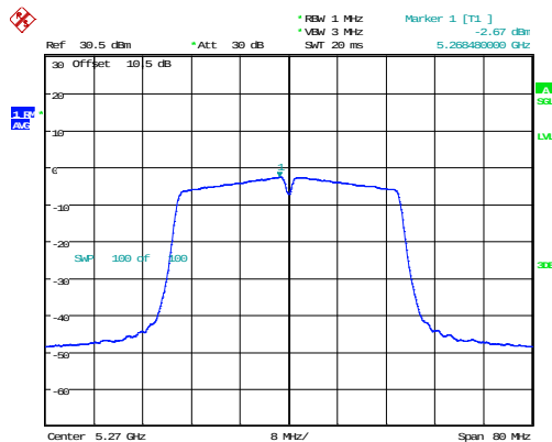
802.11n40_5270MHz_Chain 0
