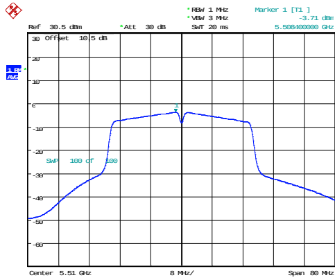
802.11n40_5510MHz_Chain 1
