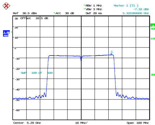
802.11ac80_5290MHz_Chain 0
