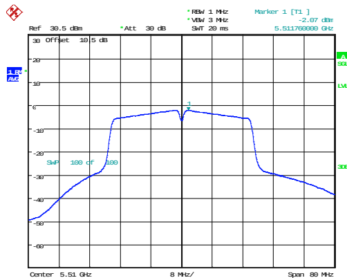
802.11n40_5510MHz_Chain 0
