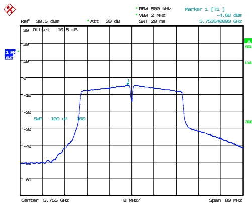
802.11n40_5755MHz_Chain 0
