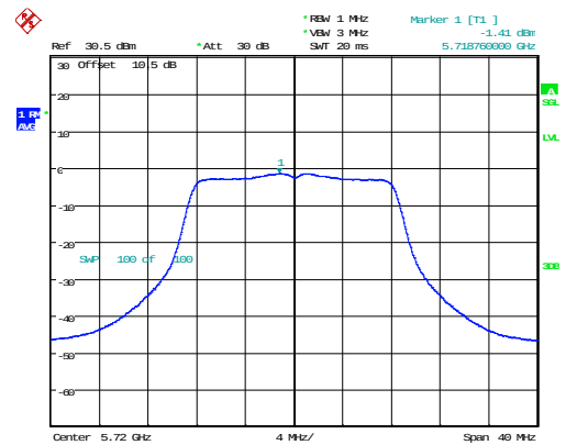
802.11a_5720MHz_Chain 1
