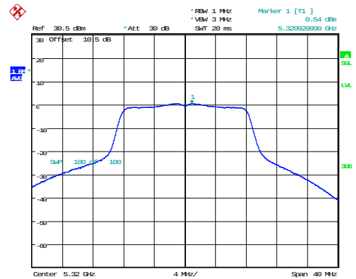
802.11a_5320MHz_Chain 1
