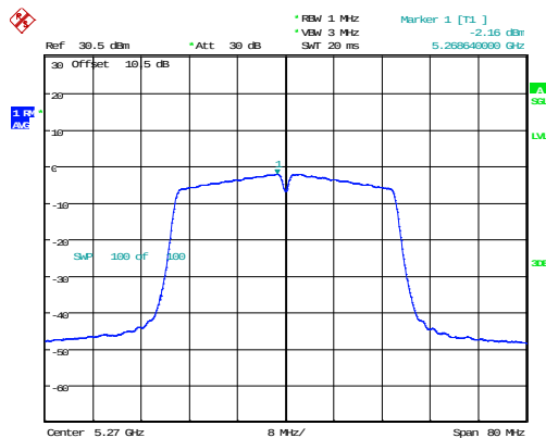
802.11n40_5270MHz_Chain 1
