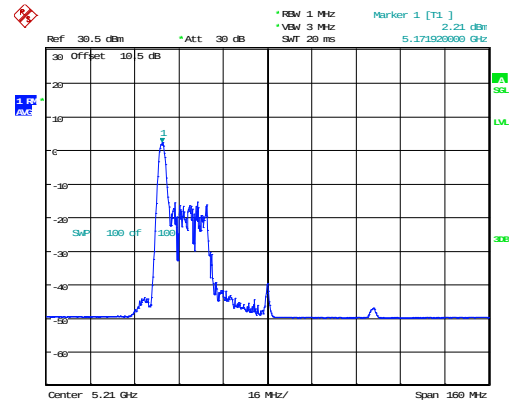
802.11ax80_5210MHz_RU_26/0_Chain 1
