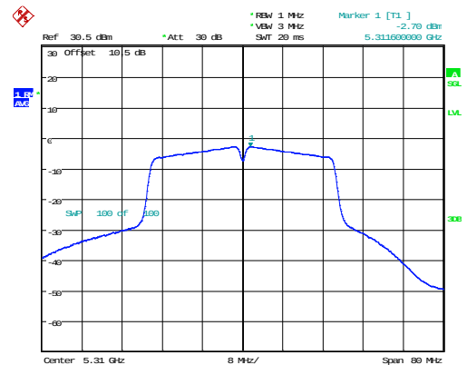
802.11n40_5310MHz_Chain 0
