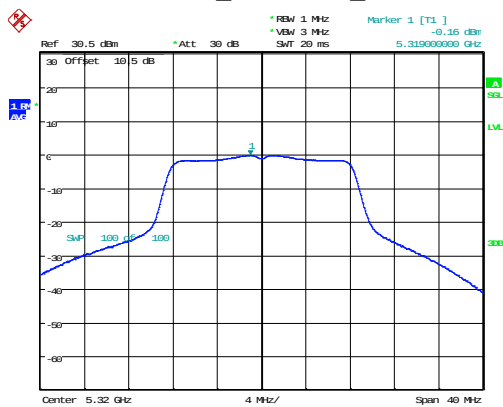
802.11a_5320MHz_Chain 0
