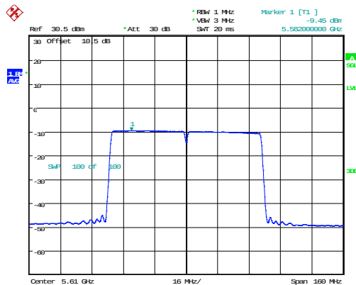
802.11ac80_5610MHz_Chain 1
