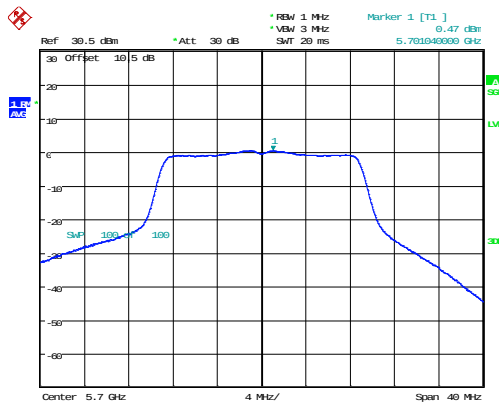
802.11n20_5700MHz_Chain 0
