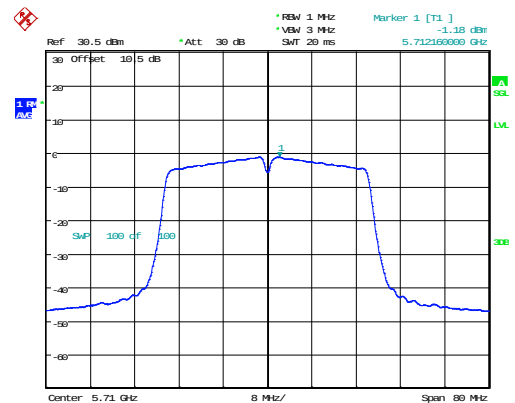
802.11n40_5710MHz_Chain 0
