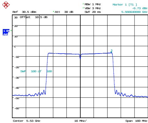
802.11ac80_5530MHz_Chain 0
