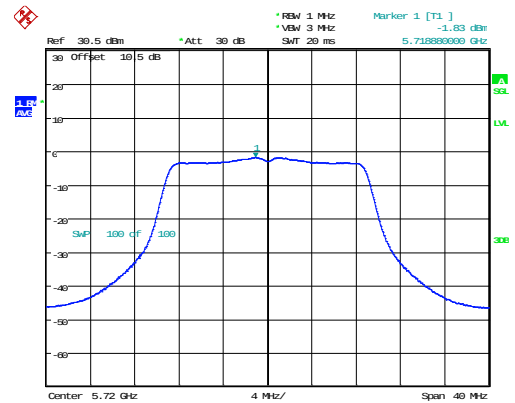
802.11n20_5720MHz_Chain 1
