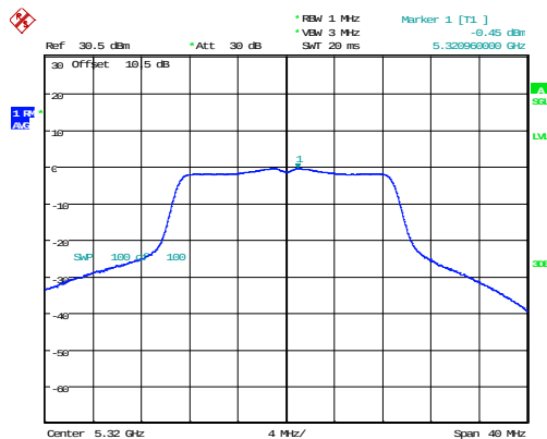
802.11n20_5320MHz_Chain 0
