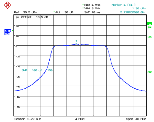
802.11a_5720MHz_Chain 0
