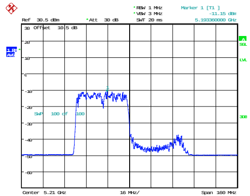
802.11ax80_5210MHz_RU_484/65_Chain 1
