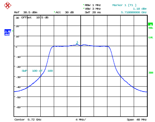
802.11n20_5720MHz_Chain 0
