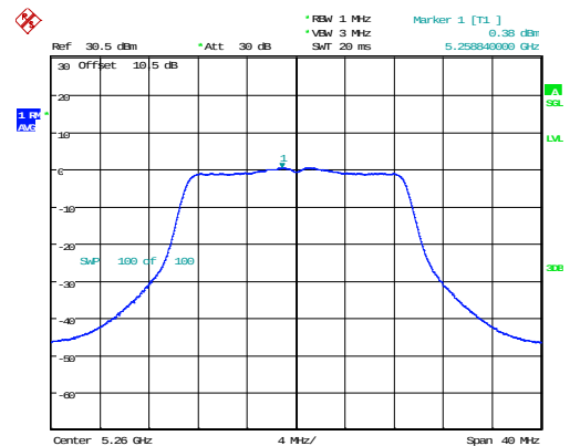
802.11n20_5260MHz_Chain 1
