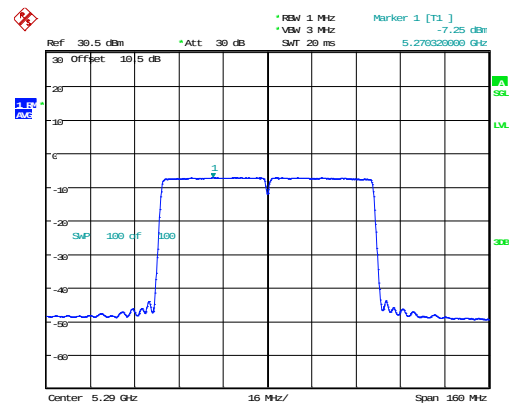
802.11ac80_5290MHz_Chain 1
