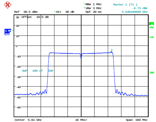
802.11ac80_5610MHz_Chain 0
