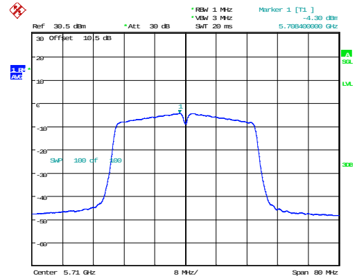
802.11n40_5710MHz_Chain 1
