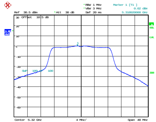
802.11n20_5320MHz_Chain 1
