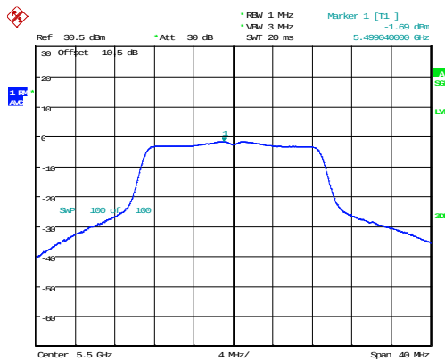
802.11n20_5500MHz_Chain 1
