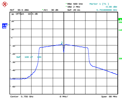
802.11n40_5755MHz_Chain 1
