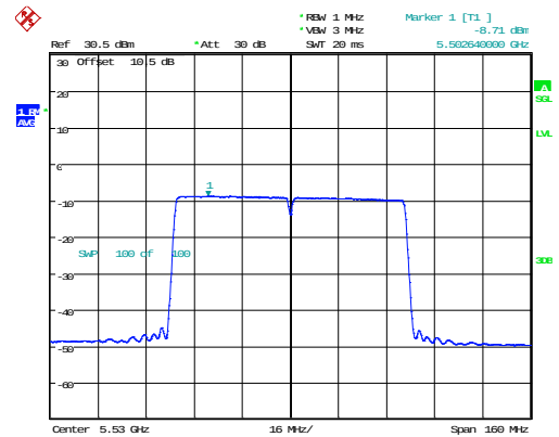
802.11ac80_5530MHz_Chain 1
