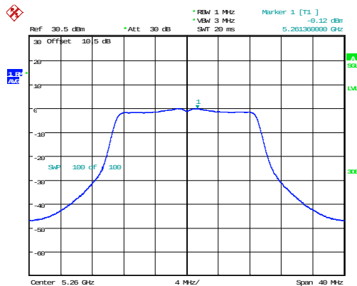
802.11n20_5260MHz_Chain 0
