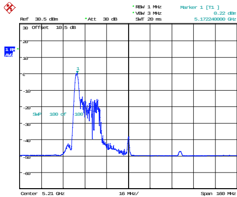
802.11ax80_5210MHz_RU_26/0_Chain 0
