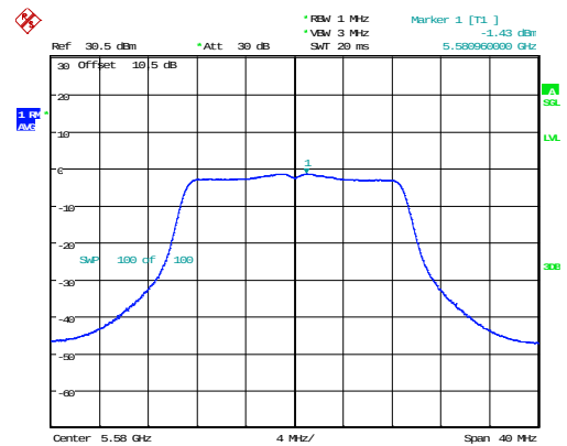
802.11n20_5580MHz_Chain 1
