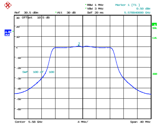
802.11n20_5580MHz_Chain 0
