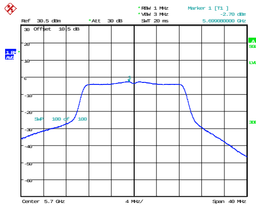
802.11n20_5700MHz_Chain 1
