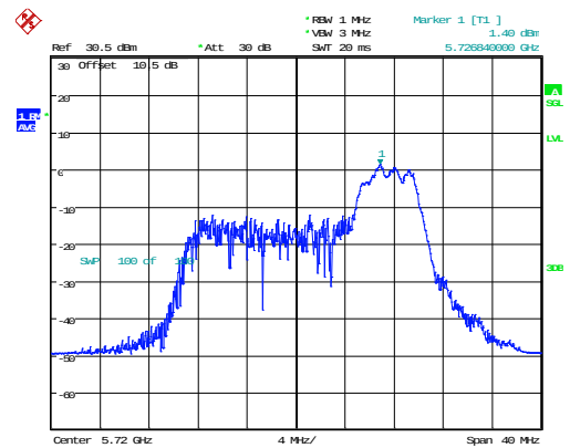
802.11ax20_5720MHz_RU_52/40_Chain 0
