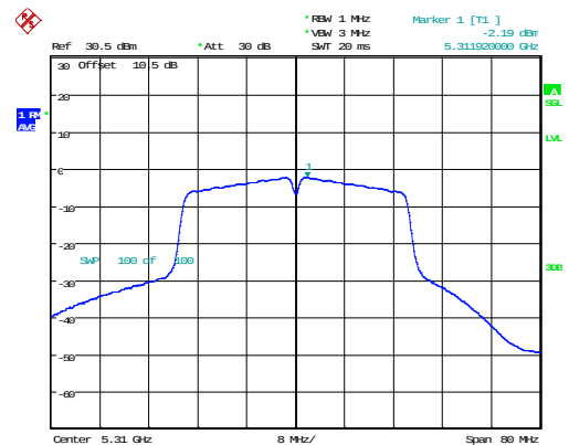
802.11n40_5310MHz_Chain 1
