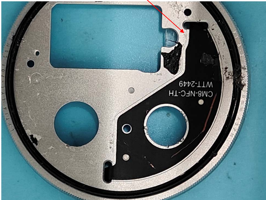
NFC Antenna
