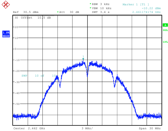
802.11b_2462MHz_Chain 1
