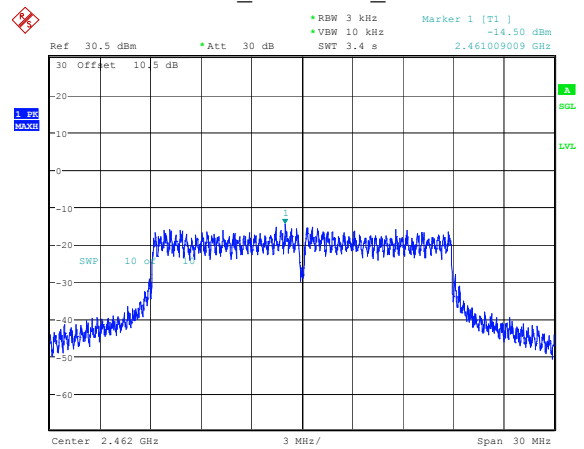
802.11n20_2462MHz_Chain 1
