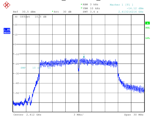
802.11n20_2412MHz_Chain 1
