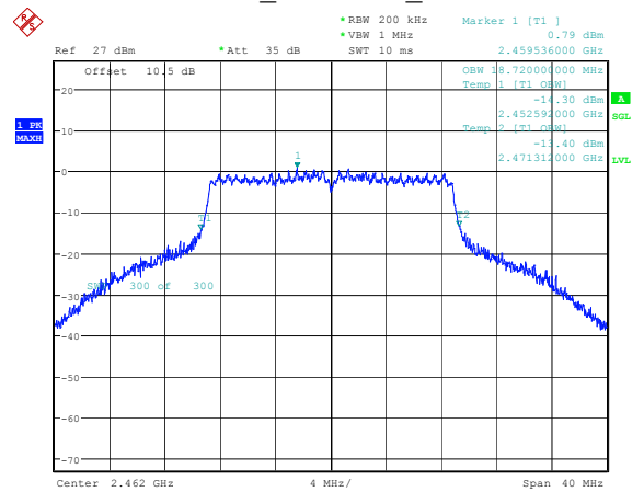
802.11n20_2462MHz_Chain 1
