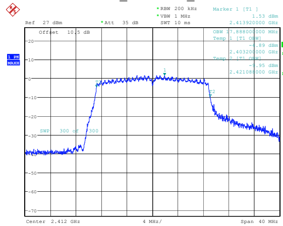
802.11n20_2412MHz_Chain 1
