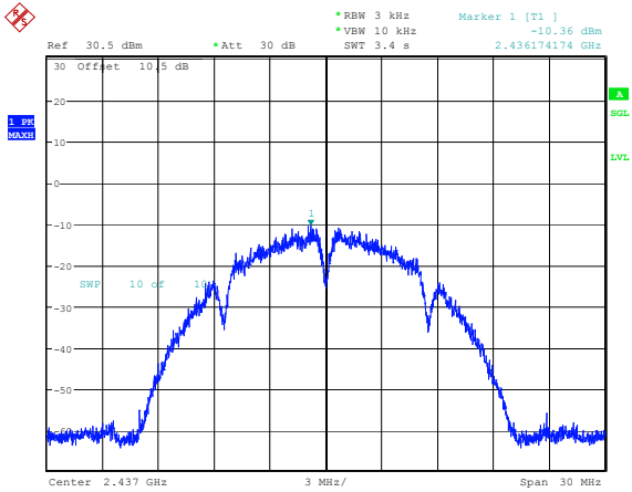
802.11b_2437MHz_Chain 1
