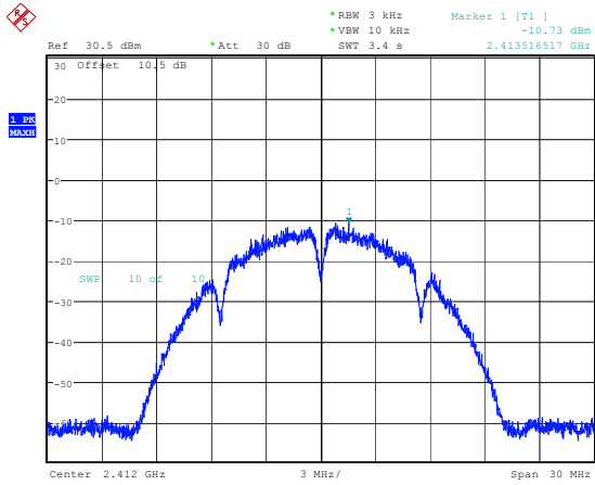
802.11b_2412MHz_Chain 1
