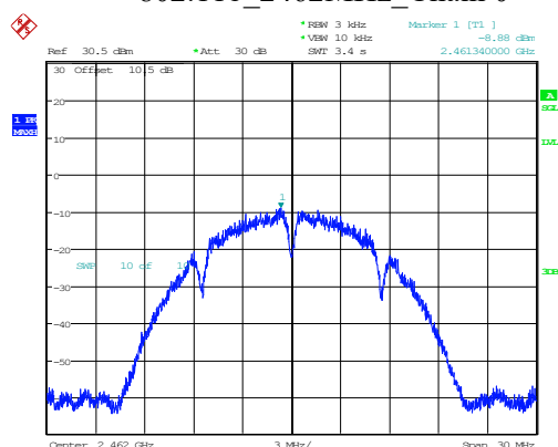
802.11b 2462MHz Chain 0
