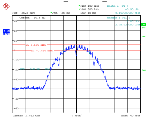
802.11b 2462MHz Chain 0
