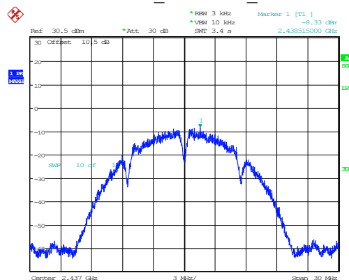
802.11b 2437MHz Chain 0
