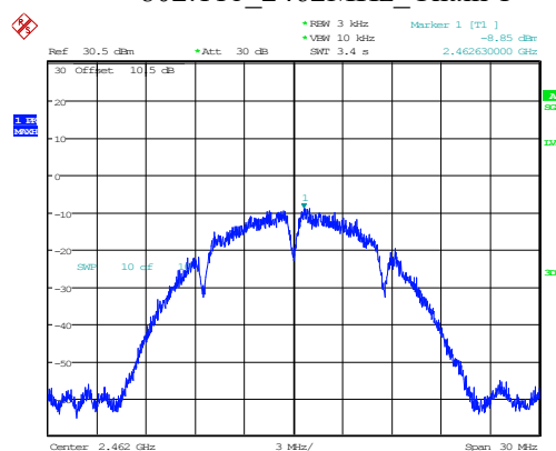
802.11b 2462MHz Chain 1
