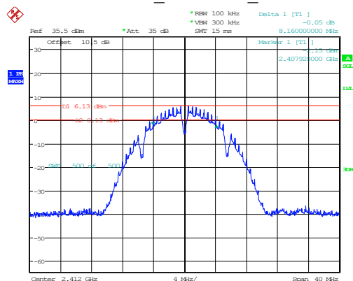
802.11b 2412MHz Chain 0
