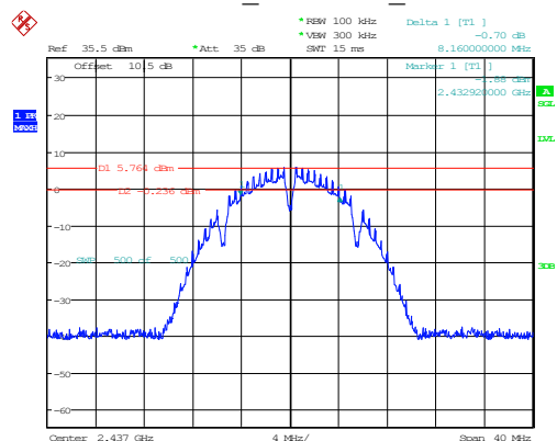
802.11b 2437MHz Chain 0
