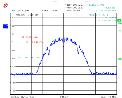
802.11b 2412MHz Chain 1
