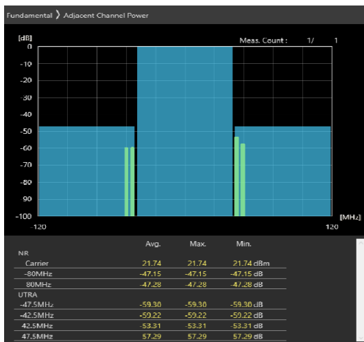
80MHz_30kHz_3660MHz-OFDM QPSK_RB1@216 -47.15,-47.28dB
