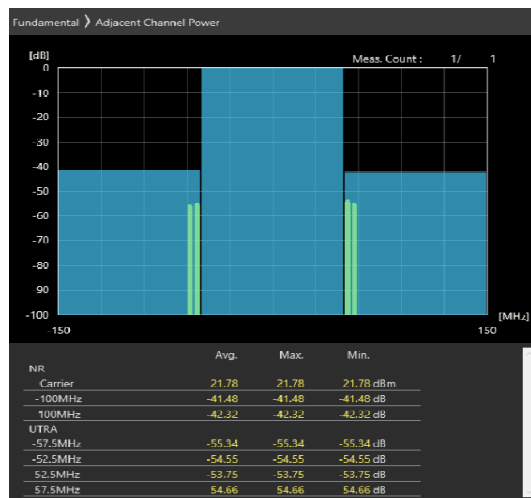
100MHz_30kHz_3650MHz-OFDM QPSK_RB270@0 -41.48,-42.32dB
