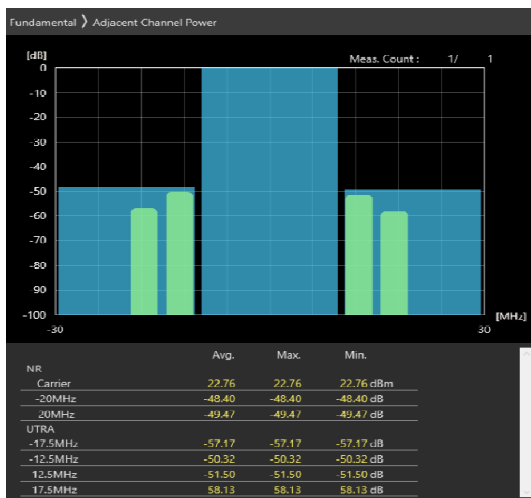
20MHz_30kHz_3690MHz-OFDM QPSK_RB25@12 -48.4,-49.47dB
