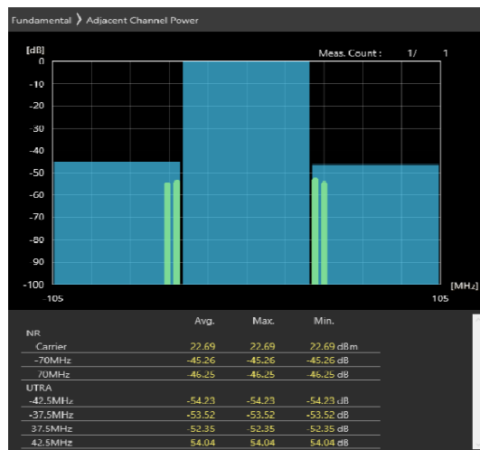
70MHz_30kHz_3665MHz-OFDM QPSK_RB90@45 -45.26,-46.25dB
