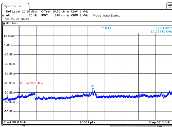
n78_2_40MHz_30kHz_3570MHz_DFT-s-OFDM QPSK_RB1@0 -47.01dBm
