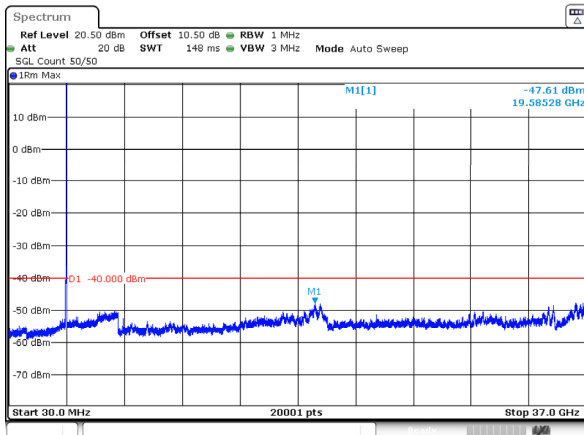
n78_2_30MHz_30kHz_3685MHz_DFT-s-OFDM QPSK_RB1@0 -47.61dBm
