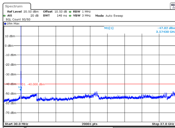
n77_2_60MHz_30kHz_3670MHz_DFT-s-OFDM QPSK_RB1@0 -47.02dBm
