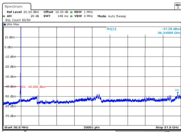
n77_2_40MHz_30kHz_3570MHz_DFT-s-OFDM QPSK_RB1@105 -47.28dBm
