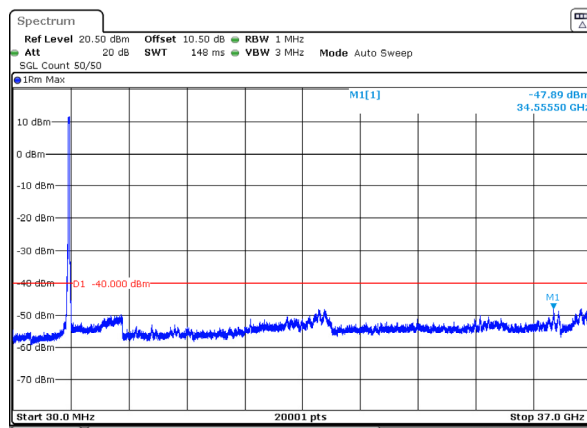
n77_2_70MHz_30kHz_3585MHz_DFT-s-OFDM QPSK_RB180@0 -47.89dBm
