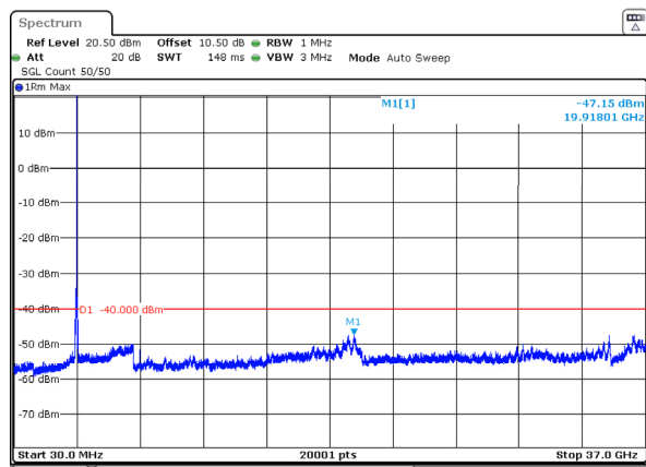
n77_2_60MHz_30kHz_3670MHz_DFT-s-OFDM QPSK_RB1@161 -47.15dBm
