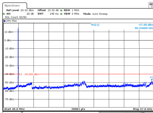
n77_2_40MHz_30kHz_3625MHz_DFT-s-OFDM QPSK_RB100@0 -47.50dBm
