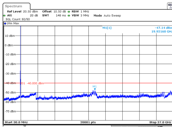
n77_2_40MHz_30kHz_3625MHz_DFT-s-OFDM QPSK_RB1@105 -47.14dBm
