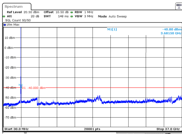
n77_2_40MHz_30kHz_3625MHz_DFT-s-OFDM QPSK_RB1@0 -40.80dBm
