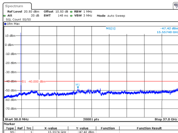
n77_2_40MHz_30kHz_3570MHz_DFT-s-OFDM QPSK_RB1@0 -47.42dBm
