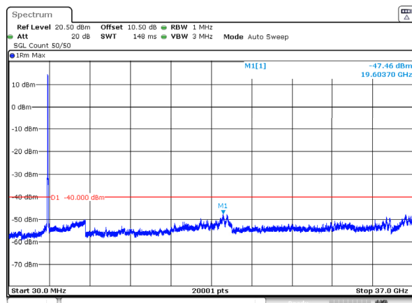
n77_2_40MHz_30kHz_3570MHz_DFT-s-OFDM QPSK_RB100@0 -47.46dBm
