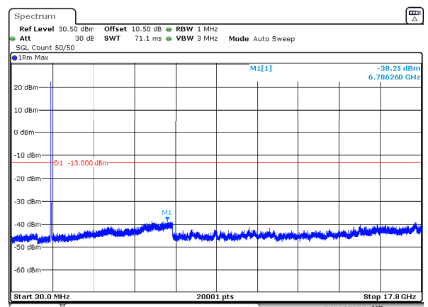
n66_20MHz_15kHz_1720MHz_DFT-s-OFDM QPSK_RB1@0 -38.25dBm
