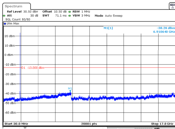
n66_15MHz_15kHz_1717.5MHz_DFT-s-OFDM QPSK_RB1@0 -38.28dBm
