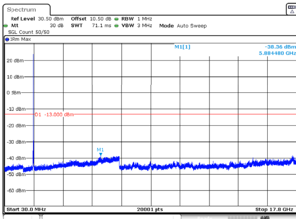
n66_25MHz_15kHz_1767.5MHz_DFT-s-OFDM QPSK_RB1@0 -38.36dBm
