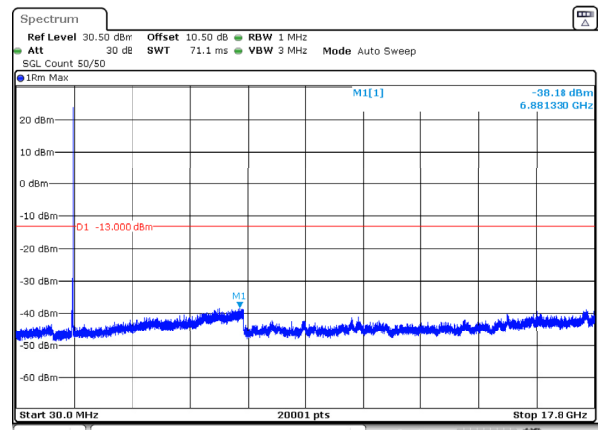
n66_20MHz_15kHz_1745MHz_DFT-s-OFDM QPSK_RB1@105 -38.18dBm
