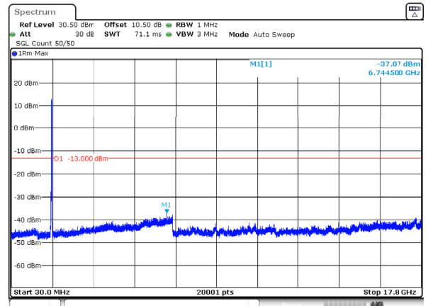
n66_20MHz_15kHz_1745MHz_DFT-s-OFDM QPSK_RB100@0 -37.07dBm
