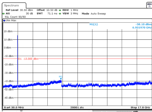
n66_10MHz_15kHz_1775MHz_DFT-s-OFDM QPSK_RB50@0 -38.10dBm
