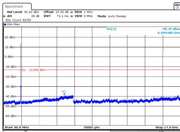
n66_15MHz_15kHz_1717.5MHz_DFT-s-OFDM QPSK_RB75@0 -38.49dBm
