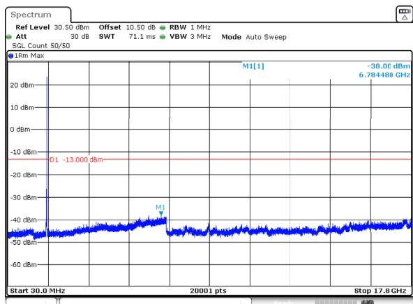
n66_25MHz_15kHz_1722.5MHz_DFT-s-OFDM QPSK_RB1@132 -38dBm
