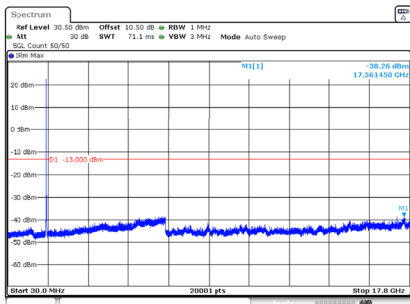
n66_25MHz_15kHz_1722.5MHz_DFT-s-OFDM QPSK_RB1@0 -38.26dBm
