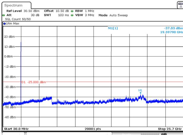
n7_5MHz_15kHz_2567.5MHz_DFT-s-OFDM QPSK_RB25@0 -37.03dBm
