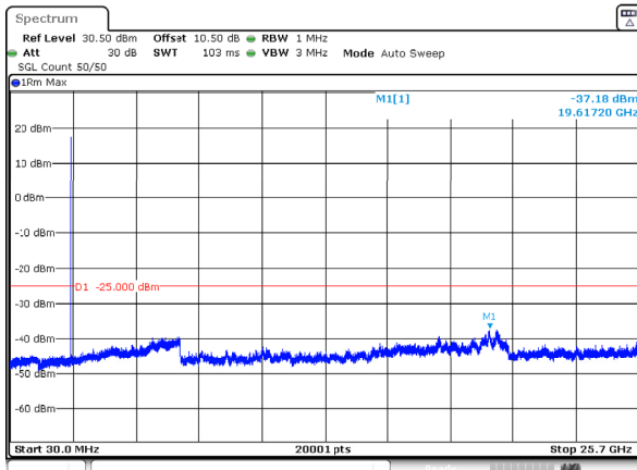
n7_10MHz_15kHz_2505MHz_DFT-s-OFDM QPSK_RB1@51 -37.18dBm
