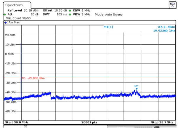
n7_10MHz_15kHz_2505MHz_DFT-s-OFDM QPSK_RB50@0 -37.11dBm
