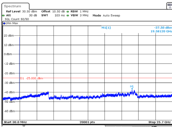
n7_10MHz_15kHz_2535MHz_DFT-s-OFDM QPSK_RB1@0 -37.50dBm
