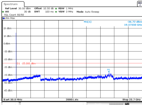
n7_5MHz_15kHz_2502.5MHz_DFT-s-OFDM QPSK_RB25@0 -36.72dBm
