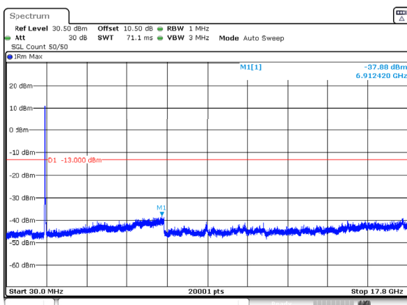
n66_30MHz_15kHz_1725MHz_DFT-s-OFDM QPSK_RB160@0 -37.88dBm
