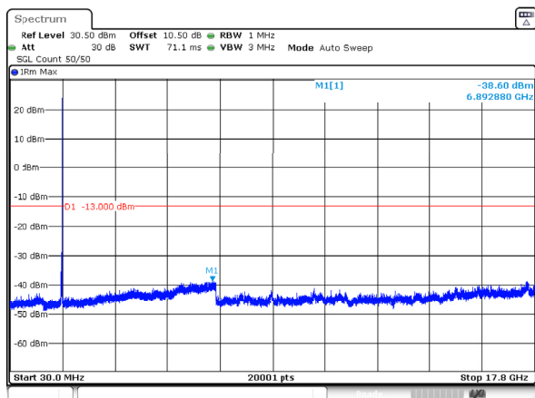
n66_20MHz_15kHz_1770MHz_DFT-s-OFDM QPSK_RB1@105 -38.60dBm
