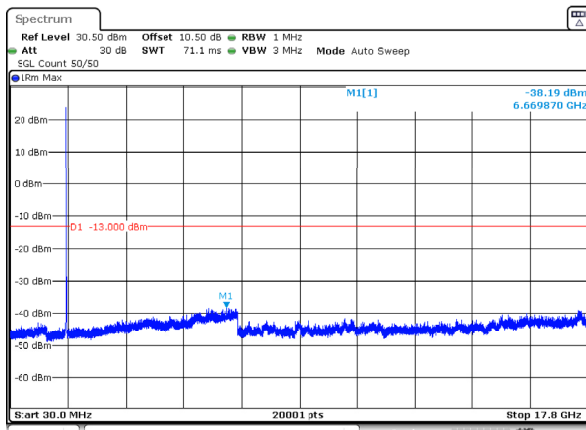
n66_20MHz_15kHz_1745MHz_DFT-s-OFDM QPSK_RB1@0 -38.19dBm
