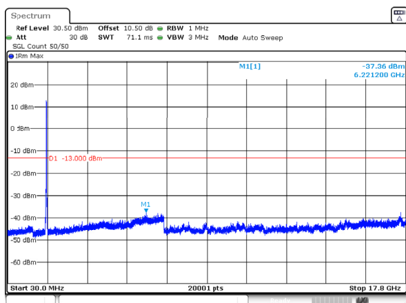
n66_25MHz_15kHz_1745MHz_DFT-s-OFDM QPSK_RB128@0 -37.36dBm
