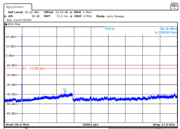
n66_20MHz_15kHz_1770MHz_DFT-s-OFDM QPSK_RB1@0 -38.18dBm
