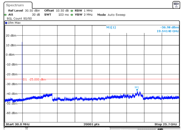
n7_5MHz_15kHz_2535MHz_DFT-s-OFDM QPSK_RB25@0 -36.90dBm
