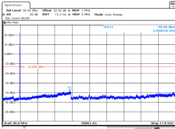
n66_20MHz_15kHz_1720MHz_DFT-s-OFDM QPSK_RB1@105 -38.08dBm
