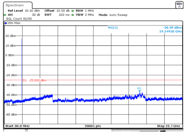
n7_10MHz_15kHz_2505MHz_DFT-s-OFDM QPSK_RB1@0 -36.99dBm
