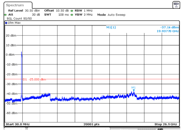
n41_100MHz_30kHz_2592.99MHz_DFT-s-OFDM QPSK_RB270@0 -37.16dBm
