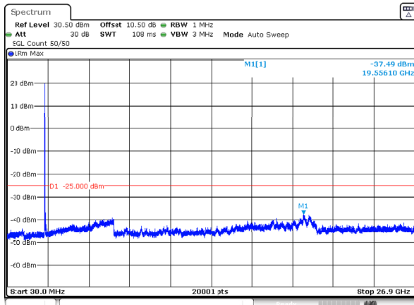
n41_40MHz_30kHz_2516.01MHz_DFT-s-OFDM QPSK_RB1@0 -37.49dBm
