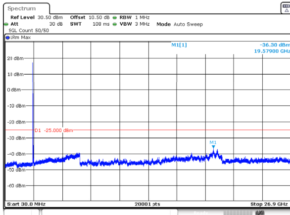
n41_60MHz_30kHz_2659.98MHz_DFT-s-OFDM QPSK_RB1@0 -36.30dBm
