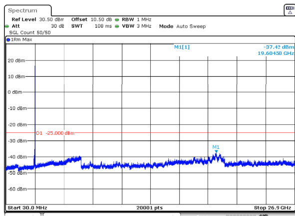
n41_80MHz_30kHz_2649.99MHz_DFT-s-OFDM QPSK_RB1@216 -37.42dBm
