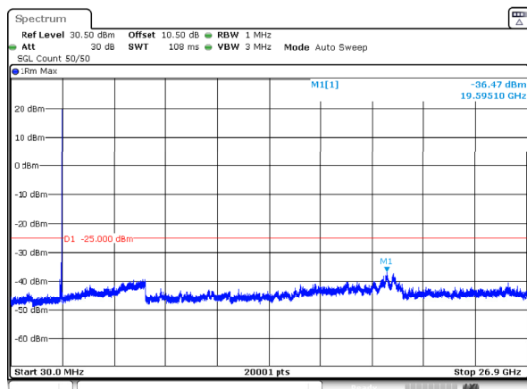
n41_90MHz_30kHz_2644.98MHz_DFT-s-OFDM QPSK_RB1@244 -36.47dBm
