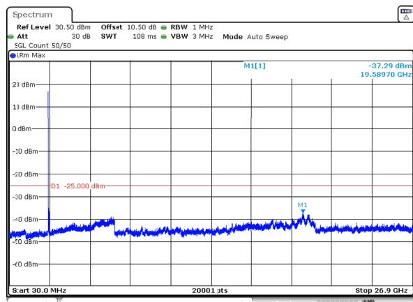
n41_80MHz_30kHz_2649.99MHz_DFT-s-OFDM QPSK_RB1@0 -37.29dBm
