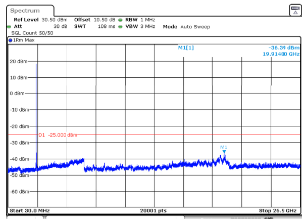
n41_40MHz_30kHz_2592.99MHz_DFT-s-OFDM QPSK_RB1@0 -36.39dBm
