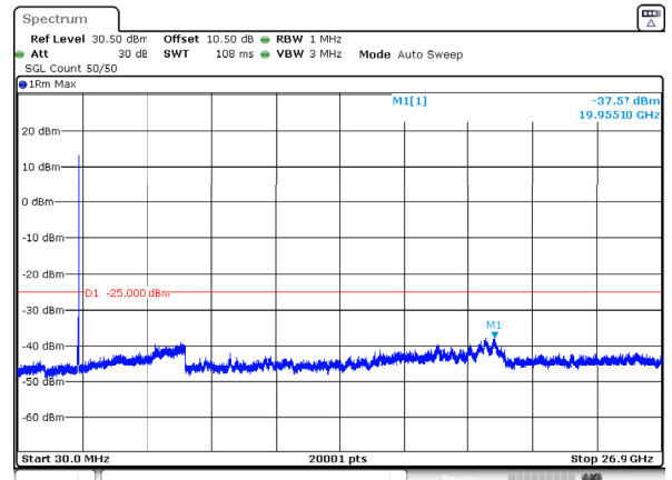
n41_40MHz_30kHz_2516.01MHz_DFT-s-OFDM QPSK_RB1@105 -37.57dBm
