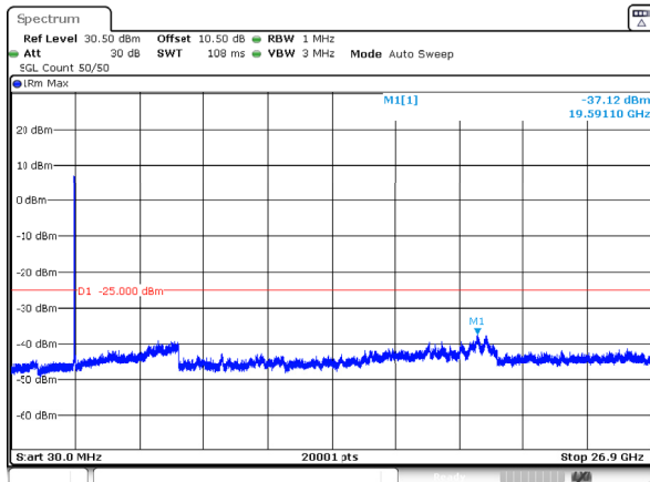
n41_30MHz_30kHz_2674.98MHz_DFT-s-OFDM QPSK_RB75@0 -37.12dBm
