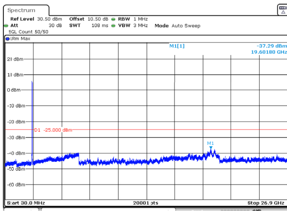
n41_40MHz_30kHz_2592.99MHz_DFT-s-OFDM QPSK_RB100@0 -37.29dBm
