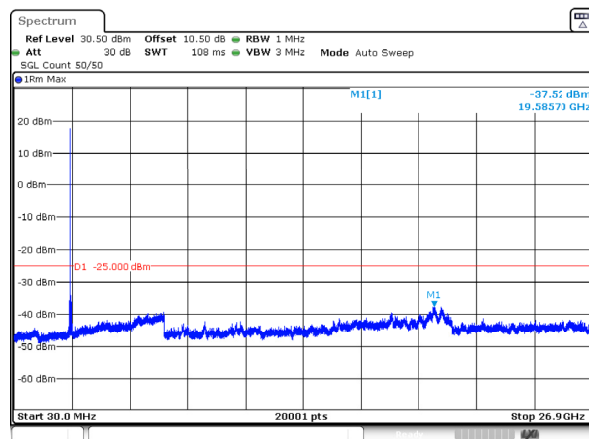
n41_90MHz_30kHz_2644.98MHz_DFT-s-OFDM QPSK_RB1@0 -37.52dBm
