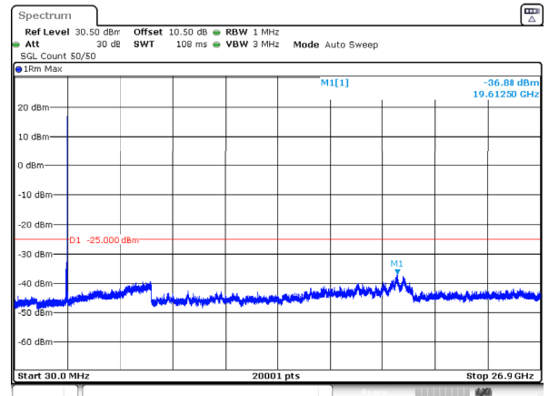
n41_60MHz_30kHz_2659.98MHz_DFT-s-OFDM QPSK_RB1@161 -36.88dBm
