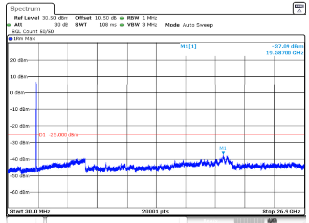
n41_40MHz_30kHz_2516.01MHz_DFT-s-OFDM QPSK_RB100@0 -37.09dBm
