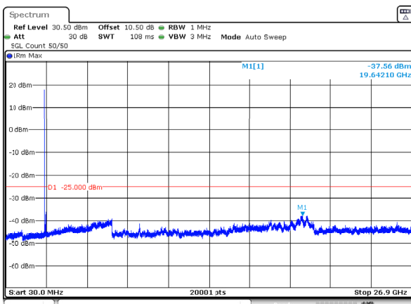
n41_100MHz_30kHz_2640MHz_DFT-s-OFDM QPSK_RB1@0 -37.56dBm
