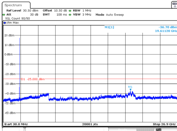
n41_50MHz_30kHz_2521.02MHz_DFT-s-OFDM QPSK_RB1@132 -36.70dBm
