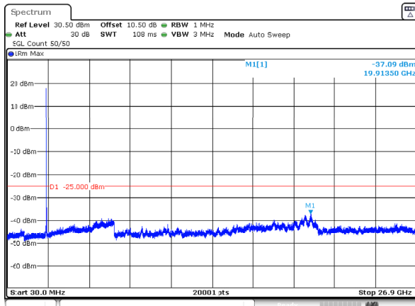
n41_50MHz_30kHz_2592.99MHz_DFT-s-OFDM QPSK_RB1@0 -37.09dBm
