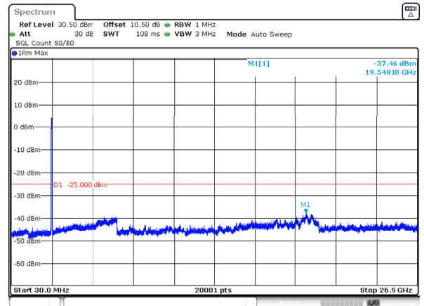
n41_60MHz_30kHz_2659.98MHz_DFT-s-OFDM QPSK_RB162@0 -37.46dBm
