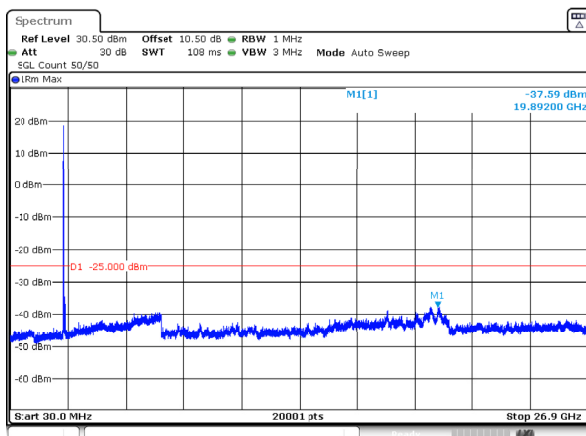
n41_80MHz_30kHz_2536.02MHz_DFT-s-OFDM QPSK_RB1@0 -37.59dBm
