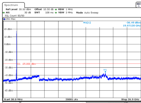
n41_80MHz_30kHz_2592.99MHz_DFT-s-OFDM QPSK_RB1@216 -36.49dBm
