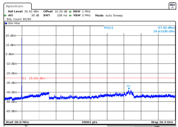
n41_50MHz_30kHz_2664.99MHz_DFT-s-OFDM QPSK_RB1@0 -37.03dBm
