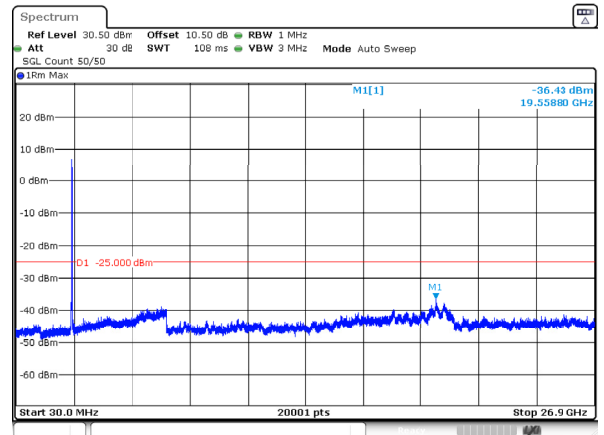
n41_50MHz_30kHz_2592.99MHz_DFT-s-OFDM QPSK_RB128@0 -36.43dBm
