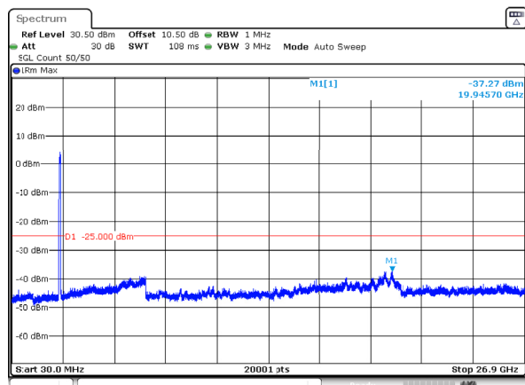
n41_80MHz_30kHz_2536.02MHz_DFT-s-OFDM QPSK_RB216@0 -37.27dBm
