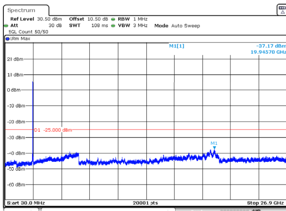
n41_50MHz_30kHz_2664.99MHz_DFT-s-OFDM QPSK_RB128@0 -37.17dBm
