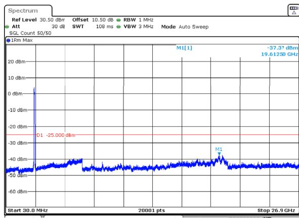
n41_80MHz_30kHz_2592.99MHz_DFT-s-OFDM QPSK_RB216@0 -37.37dBm
