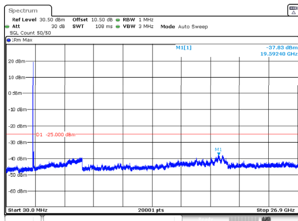
n41_100MHz_30kHz_2546.01MHz_DFT-s-OFDM QPSK_RB1@0 -37.83dBm
