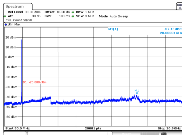
n41_100MHz_30kHz_2546.01MHz_DFT-s-OFDM QPSK_RB1@272 -37.16dBm
