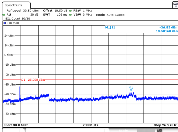
n41_60MHz_30kHz_2592.99MHz_DFT-s-OFDM QPSK_RB1@161 -36.85dBm
