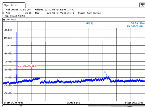
n41_80MHz_30kHz_2592.99MHz_DFT-s-OFDM QPSK_RB1@0 -36.98dBm
