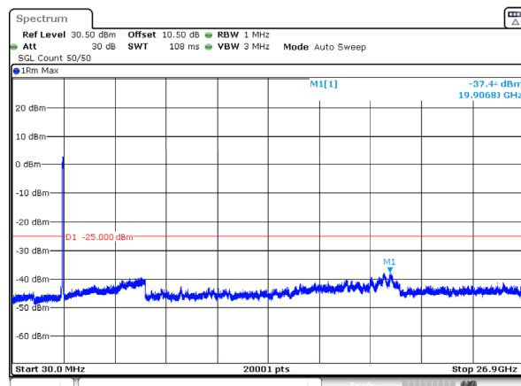
n41_90MHz_30kHz_2644.98MHz_DFT-s-OFDM QPSK_RB243@0 -37.44dBm
