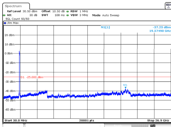
n41_90MHz_30kHz_2592.99MHz_DFT-s-OFDM QPSK_RB243@0 -37.25dBm
