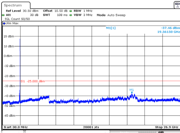
n41_100MHz_30kHz_2592.99MHz_DFT-s-OFDM QPSK_RB1@272 -37.46dBm
