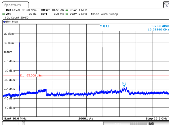
n41_15MHz_30kHz_2682.48MHz_DFT-s-OFDM QPSK_RB36@0 -37.36dBm
