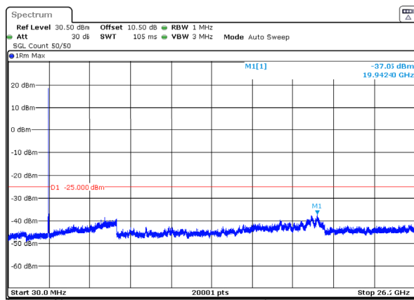
n38_40MHz_30kHz_2590MHz_DFT-s-OFDM QPSK_RB1@0 -37.05dBm
