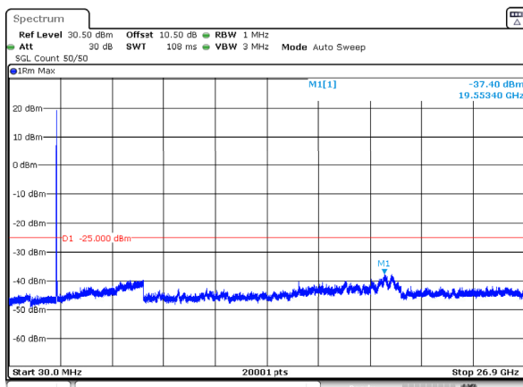
n41_30MHz_30kHz_2511MHz_DFT-s-OFDM QPSK_RB1@0 -37.40dBm
