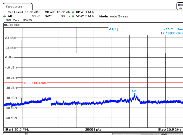
n41_15MHz_30kHz_2592.99MHz_DFT-s-OFDM QPSK_RB1@0 -36.71dBm
