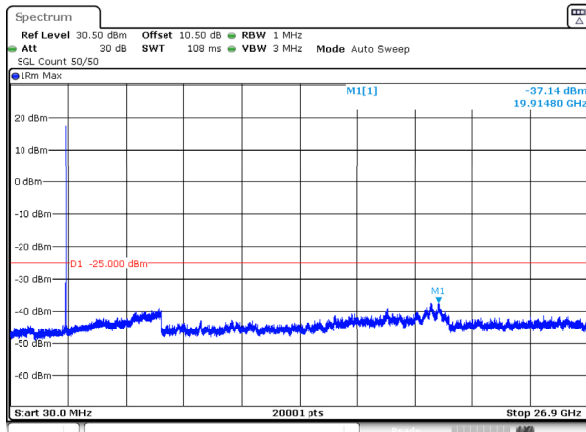
n41_30MHz_30kHz_2592.99MHz_DFT-s-OFDM QPSK_RB1@77 -37.14dBm
