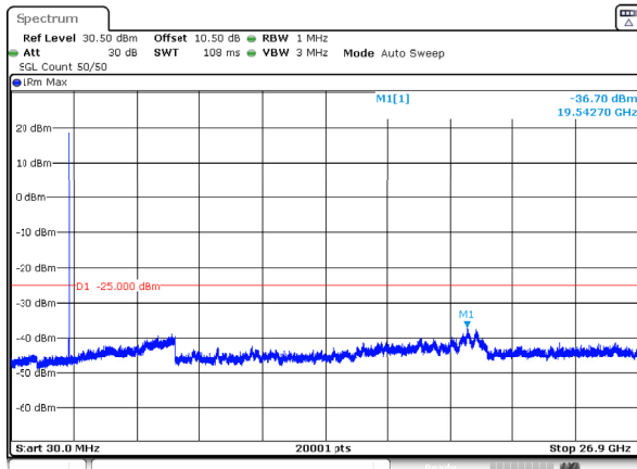
n41_20MHz_30kHz_2506.02MHz_DFT-s-OFDM QPSK_RB1@50 -36.70dBm
