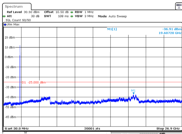
n41_15MHz_30kHz_2503.5MHz_DFT-s-OFDM QPSK_RB36@0 -36.91dBm
