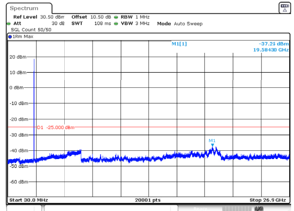
n41_20MHz_30kHz_2506.02MHz_DFT-s-OFDM QPSK_RB1@0 -37.25dBm
