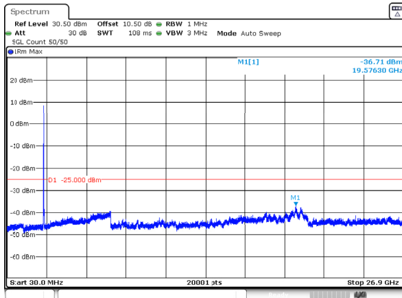
n41_30MHz_30kHz_2511MHz_DFT-s-OFDM QPSK_RB75@0 -36.71dBm
