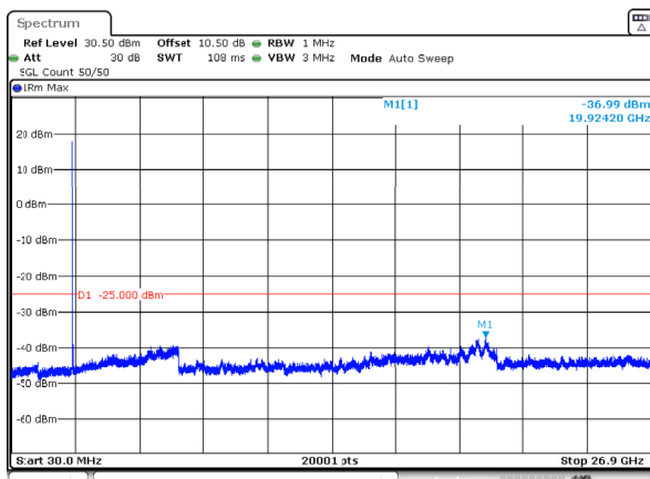
n41_20MHz_30kHz_2592.99MHz_DFT-s-OFDM QPSK_RB1@0 -36.99dBm
