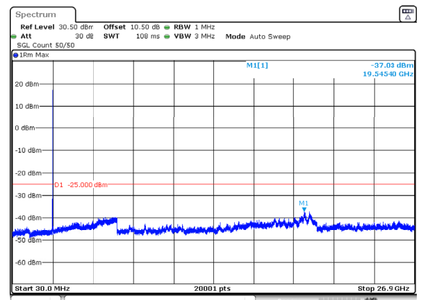
n41_30MHz_30kHz_2674.98MHz_DFT-s-OFDM QPSK_RB1@77 -37.03dBm
