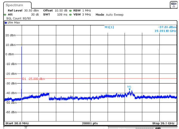
n41_20MHz_30kHz_2679.99MHz_DFT-s-OFDM QPSK_RB50@0 -37dBm
