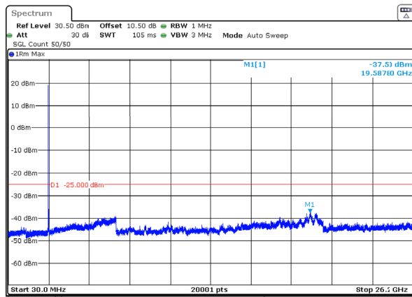
n38_30MHz_30kHz_2605MHz_DFT-s-OFDM QPSK_RB1@0 -37.50dBm
