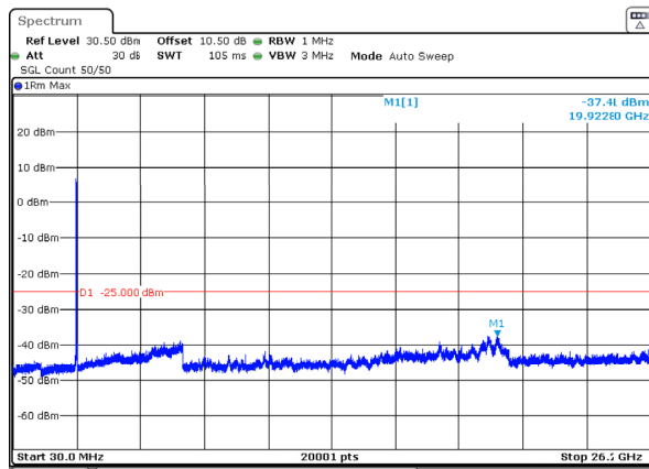
n38_30MHz_30kHz_2605MHz_DFT-s-OFDM QPSK_RB75@0 -37.41dBm
