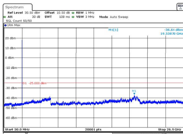
n41_15MHz_30kHz_2682.48MHz_DFT-s-OFDM QPSK_RB1@37 -36.64dBm
