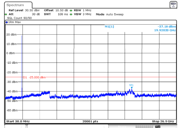
n41_30MHz_30kHz_2592.99MHz_DFT-s-OFDM QPSK_RB1@0 -37.10dBm
