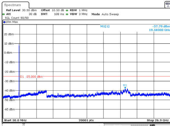
n41_20MHz_30kHz_2592.99MHz_DFT-s-OFDM QPSK_RB50@0 -37.79dBm
