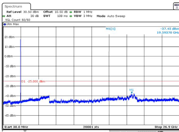
n41_30MHz_30kHz_2674.98MHz_DFT-s-OFDM QPSK_RB1@0 -37.45dBm
