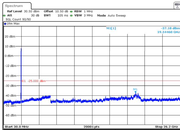
n38_30MHz_30kHz_2595MHz_DFT-s-OFDM QPSK_RB75@0 -37.18dBm
