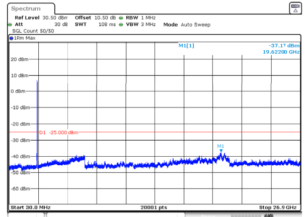
n41_30MHz_30kHz_2592.99MHz_DFT-s-OFDM QPSK_RB75@0 -37.17dBm
