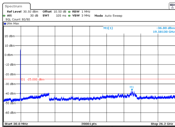
n38_40MHz_30kHz_2590MHz_DFT-s-OFDM QPSK_RB100@0 -36.80dBm
