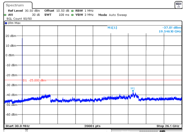
n41_20MHz_30kHz_2679.99MHz_DFT-s-OFDM QPSK_RB1@0 -37.02dBm
