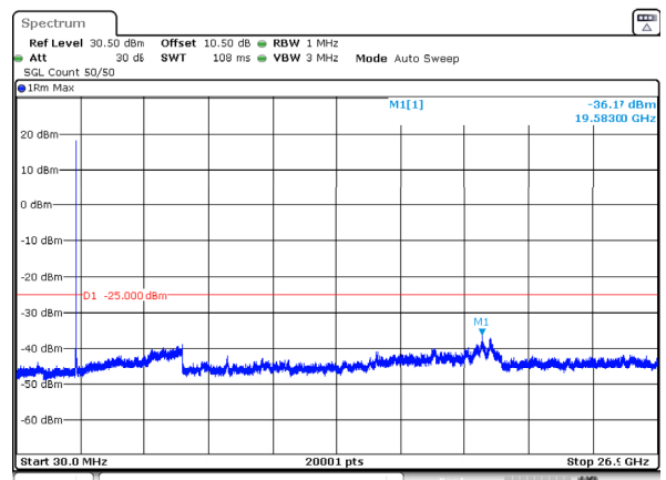
n41_30MHz_30kHz_2511MHz_DFT-s-OFDM QPSK_RB1@77 -36.17dBm
