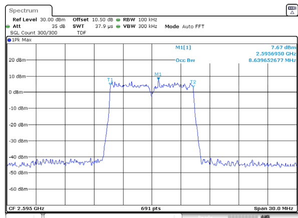
n38_10MHz_30kHz_2595MHz_DFT-s-OFDM 64 QAM_RB24@0
