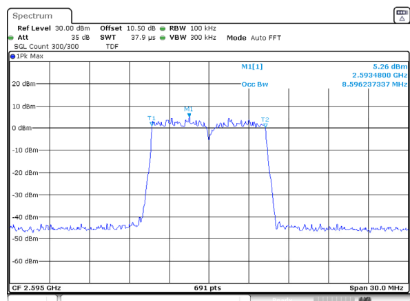
n38_10MHz_30kHz_2595MHz_DFT-s-OFDM 256 QAM_RB24@0
