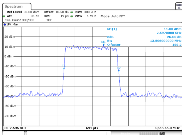
n38_15MHz_30kHz_2595MHz_DFT-s-OFDM QPSK_RB36@0
