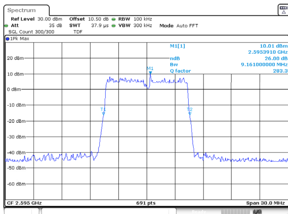
n38_10MHz_30kHz_2595MHz_DFT-s-OFDM QPSK_RB24@0
