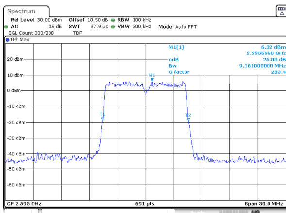
n38_10MHz_30kHz_2595MHz_DFT-s-OFDM 64 QAM_RB24@0
