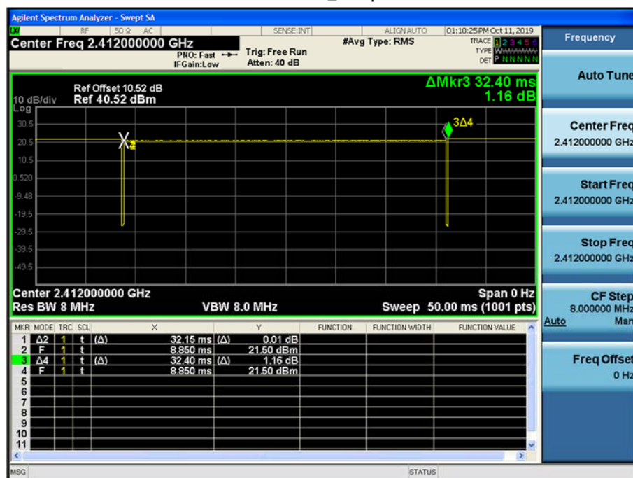
802.11b_1Mbps
