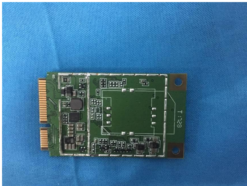
WiFi Module
