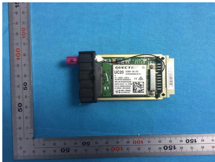
UC20(3G)
