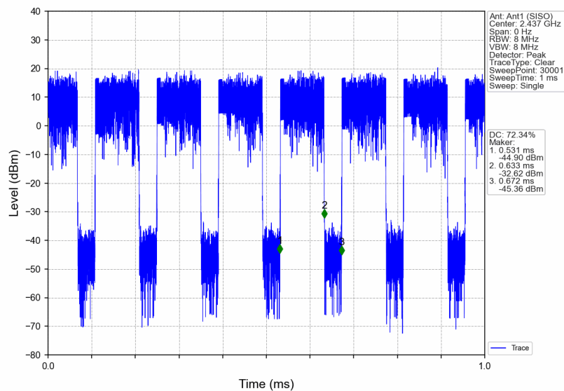
802.11n(HT20)_MCH_2437MHz_Ant1 (SISO)_NTNW
