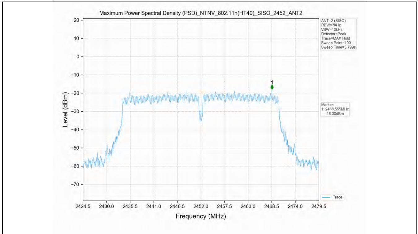
802.11n(HT40)_2452MHz_SISO_ANT2
