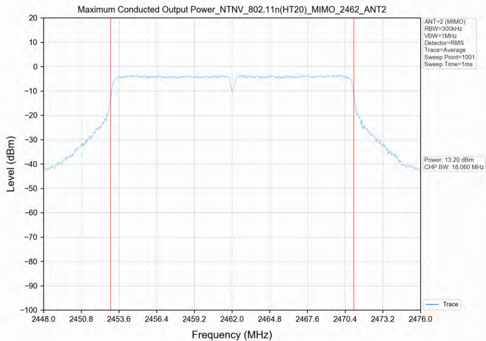
802.11n(HT20)_2462MHz_MIMO_ANT2
