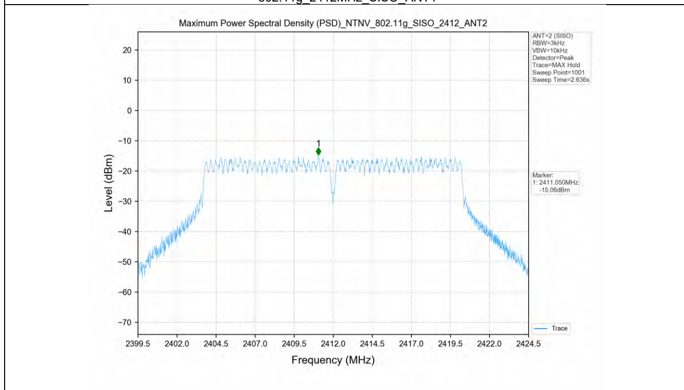
802.11g_2412MHz_SISO_ANT2
