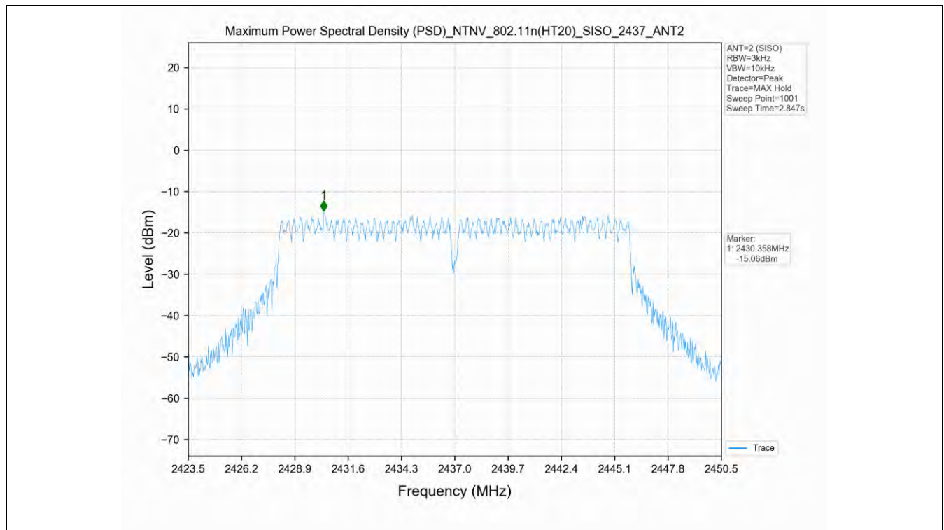
802.11n(HT20)_2437MHz_SISO_ANT2
