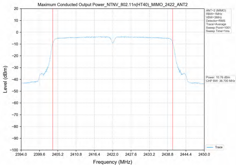
802.11n(HT40)_2422MHz_MIMO_ANT2
