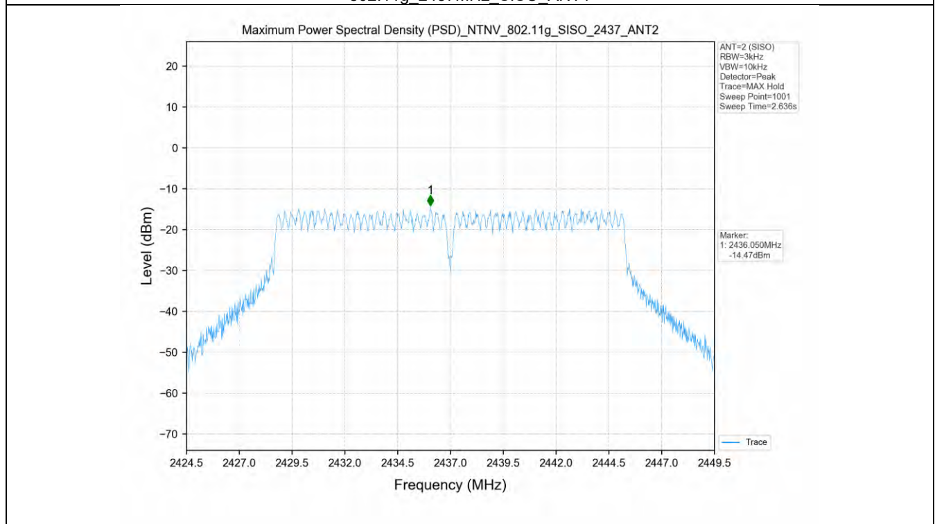
802.11g_2437MHz_SISO_ANT2
