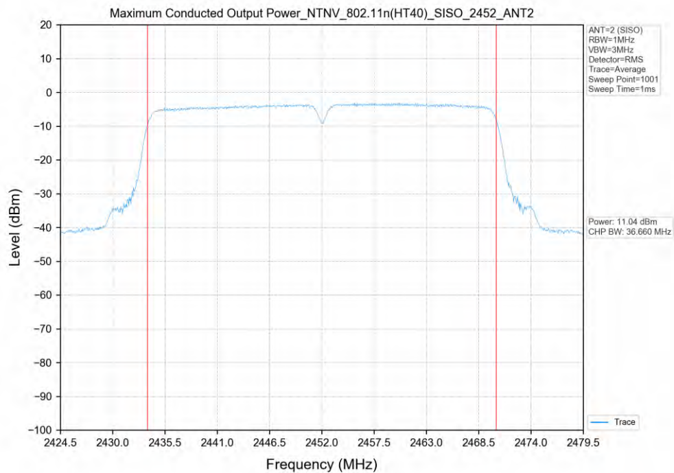
802.11n(HT40)_2452MHz_SISO_ANT2
