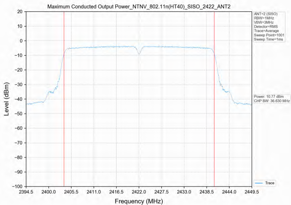
802.11n(HT40)_2422MHz_SISO_ANT2
