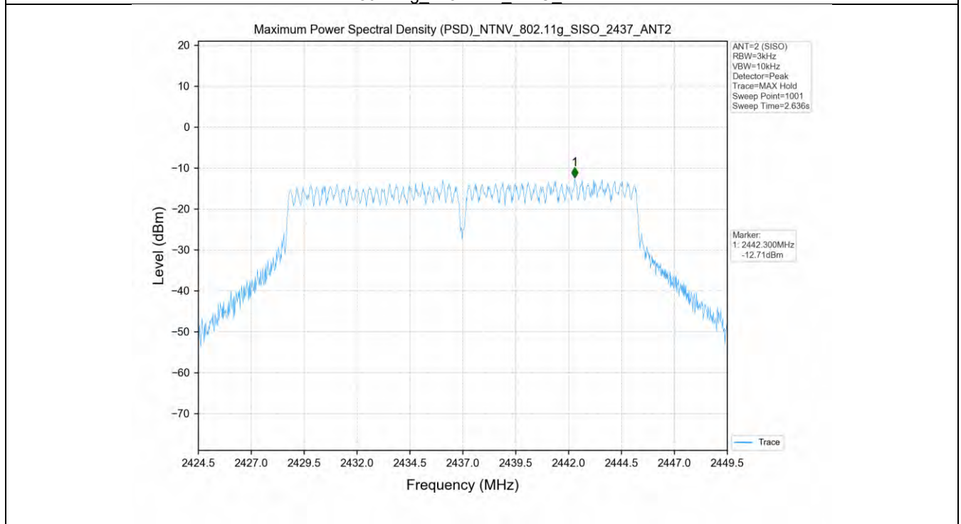
802.11g_2437MHz_SISO_ANT2
