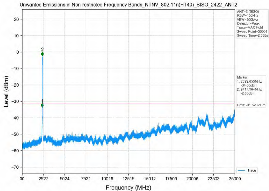
802.11n(HT40)_2422MHz_SISO_ANT2
