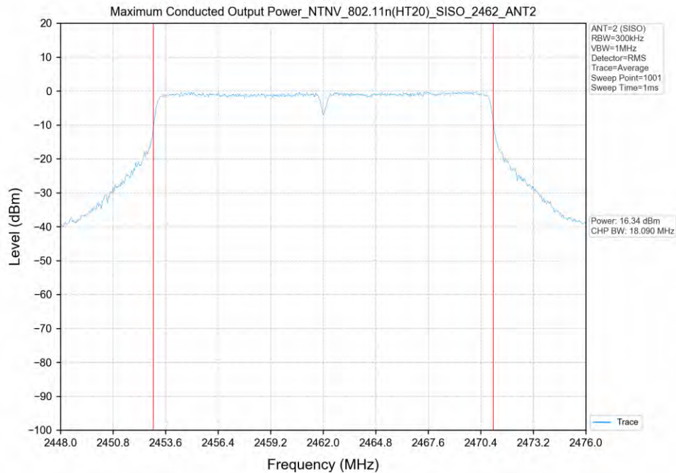
802.11n(HT20)_2462MHz_SISO_ANT2
