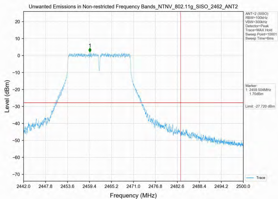
802.11g_2462MHz_SISO_ANT2
