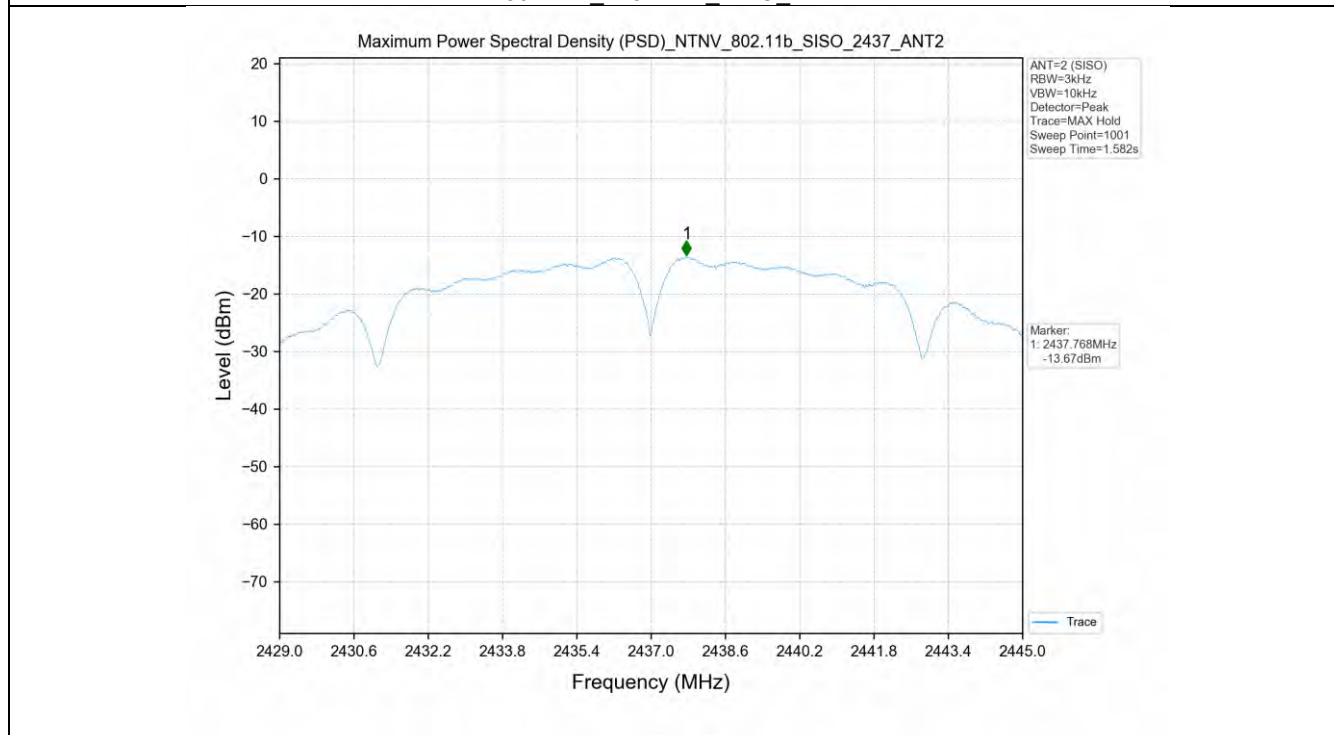
802.11b_2437MHz_SISO_ANT2
