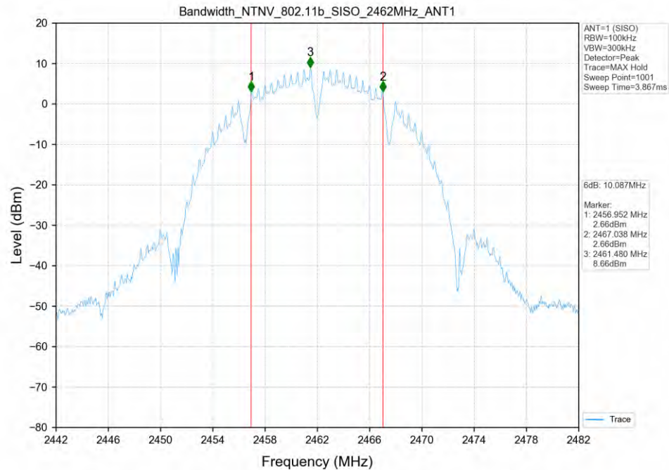
802.11b_2462MHz_SISO_ANT1
