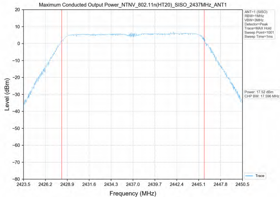
802.11n(HT20)_2437MHz_SISO_ANT1
