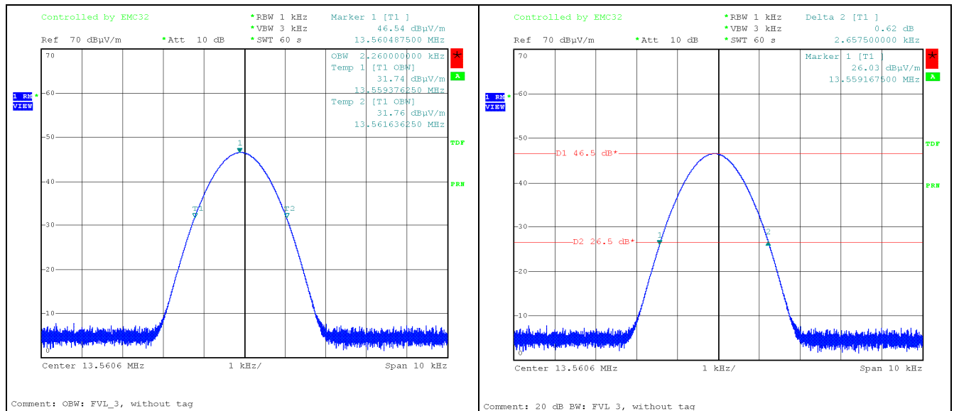
Diagram 15: 20 dB bandwidth and 99 % bandwidth at 13.56 MHz: without RFID tag [20 dB Bandbreite und 99 % Bandbreite bei 13,56 MHz: ohne RFID- Tag]
