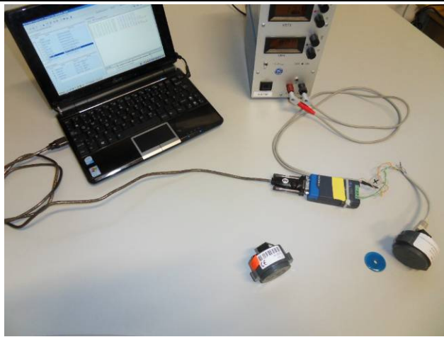
Figure 1: Test setup with unmodified sample [Prüfaufbau mit unmodifizierten Prüfmuster]
