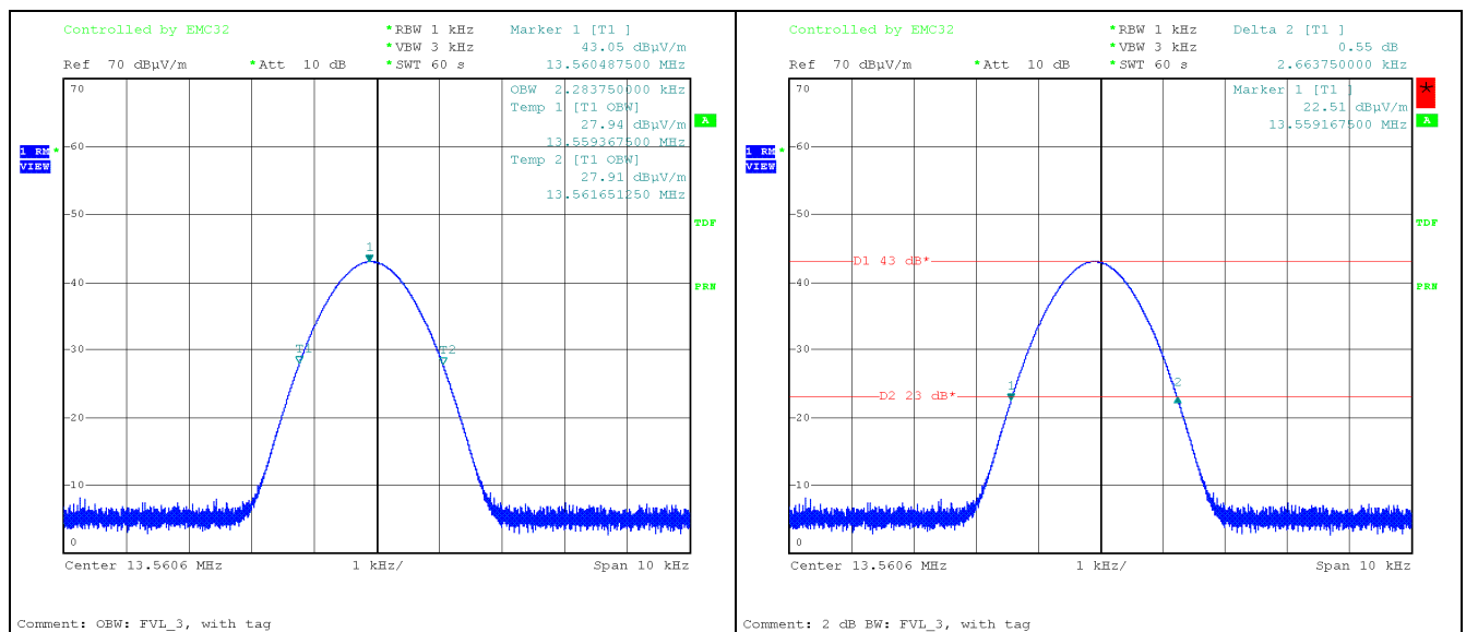
Diagram 16: 20 dB bandwidth and 99 % bandwidth at 13.56 MHz: with placed RFID tag [20 dB Bandbreite und 99 % Bandbreite bei 13,56 MHz: mit aufgelegten RFID- Tag]
