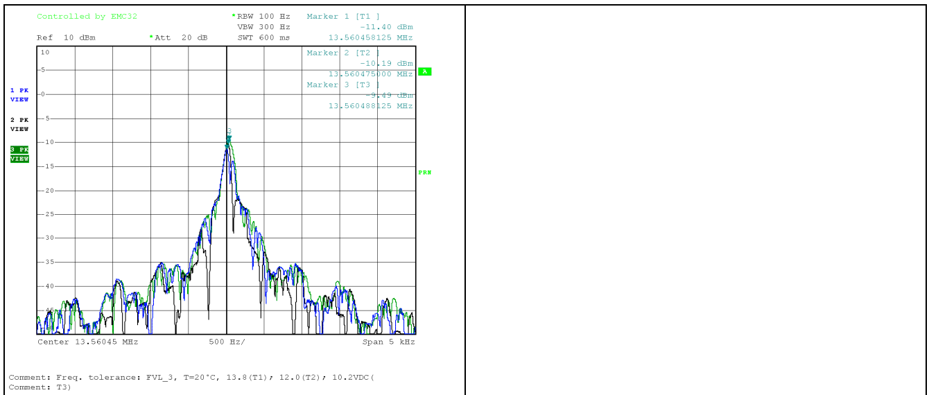
Diagram 14: Frequency tolerance at 13.56 MHz: 13.8, 12.0 and 10.2 VDC [Frequenzabweichung bei 13,56 MHz: 13,8, 12,0 und 10,2 VDC]
