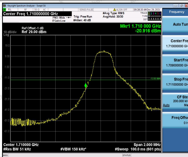
Band4-3MHz-QPSK-19965-1RB#14
