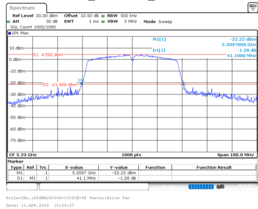
n40_5230MHz_Chain 0
