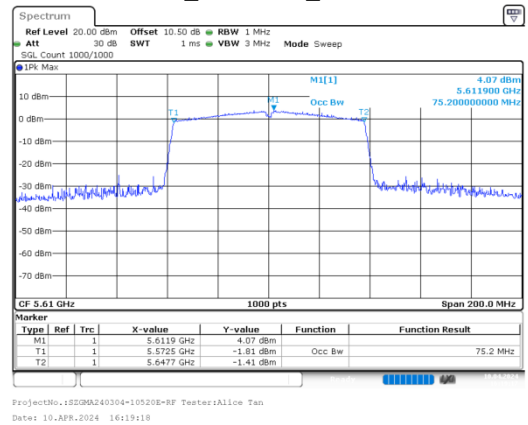
ac80_5610MHz_Chain 0
