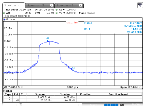
n20_2462MHz_Chain 0
