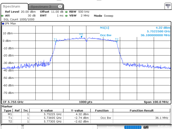
n40_5755MHz_Chain 0
