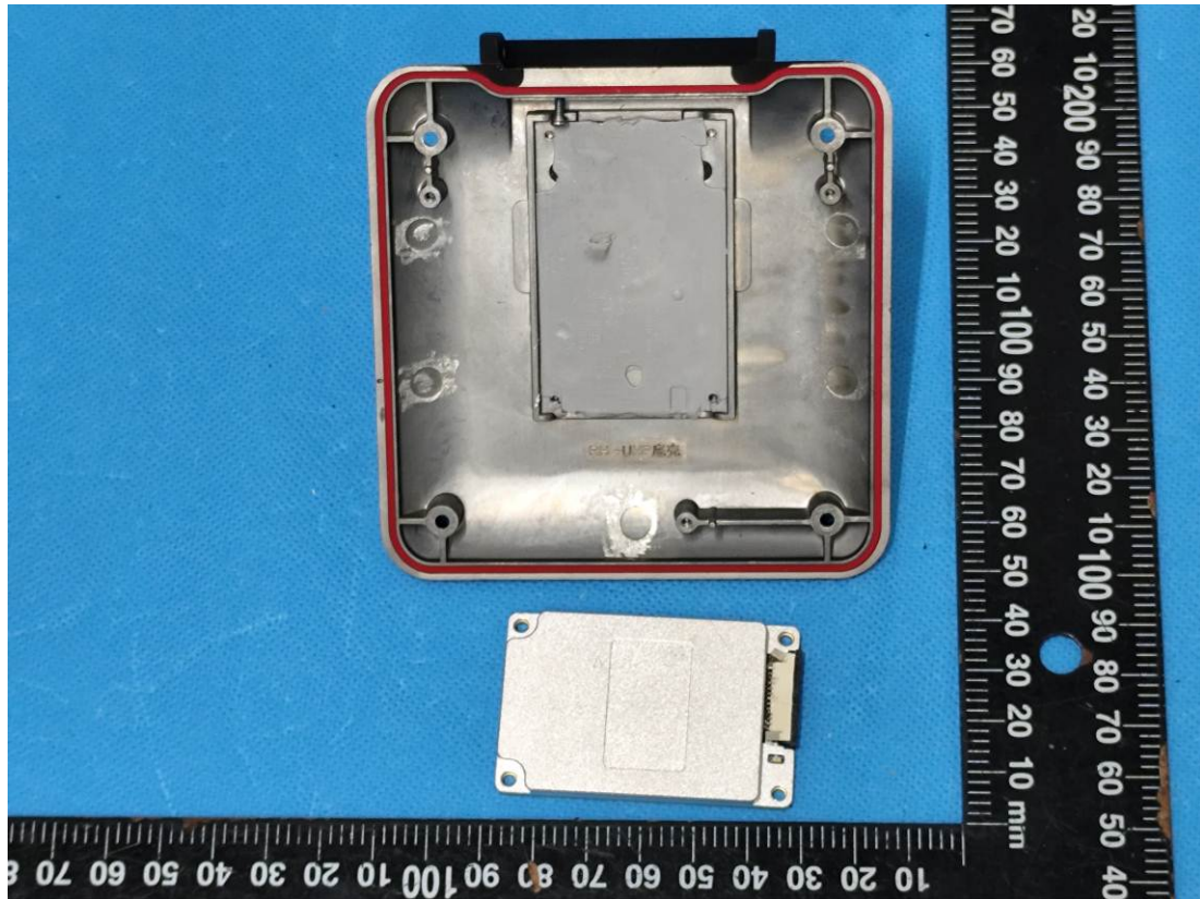
RFID Module
