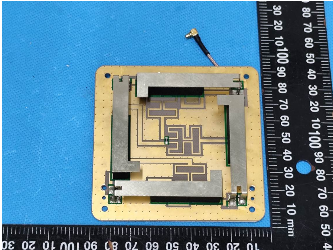
RFID Antenna
