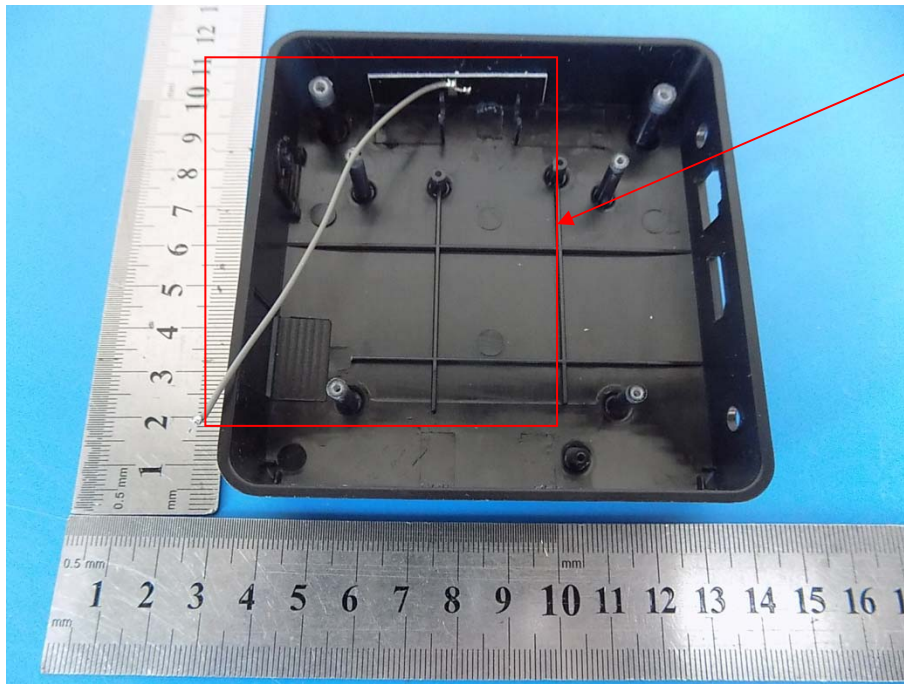
BT/WiFi Antenna
