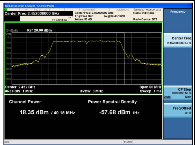
802.11n40 - AV Output power - CH 9
