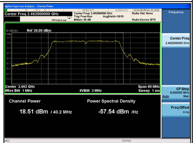
802.11n40 - AV Output power - CH 11
