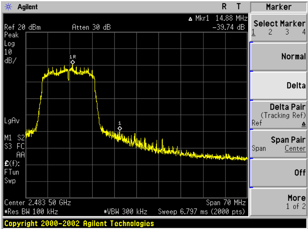
802.11g-CH11
