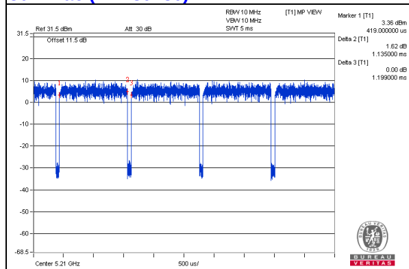
802.11ac (VHT80+80)
