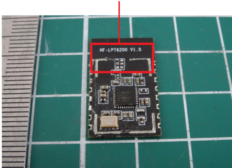
Antenna
