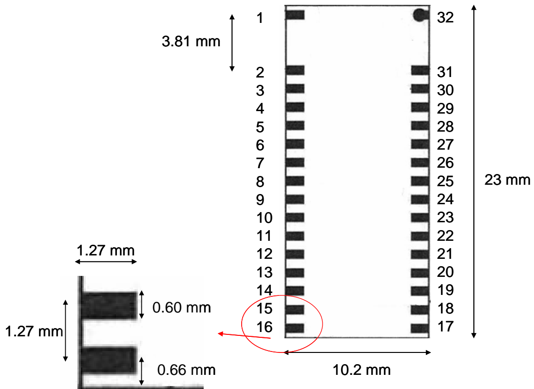
XBT40A module PIN Def
