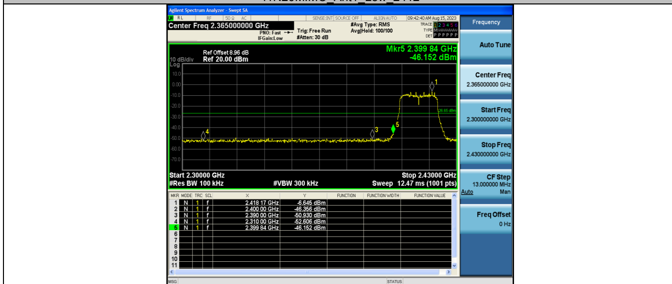
11N20MIMO_Ant2_Low_2412
