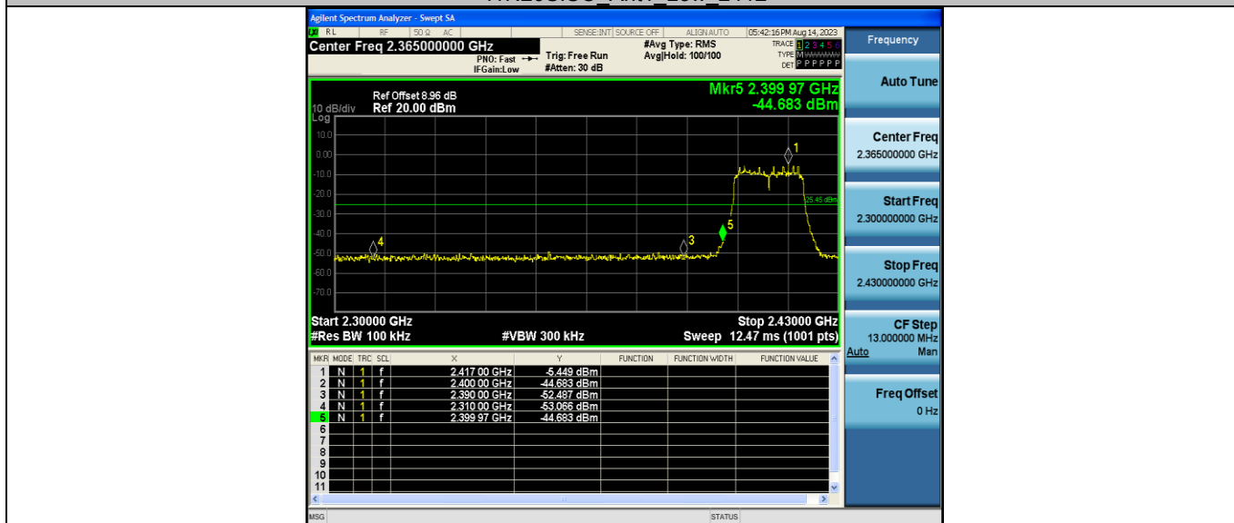
11N20SISO_Ant2_Low_2412
