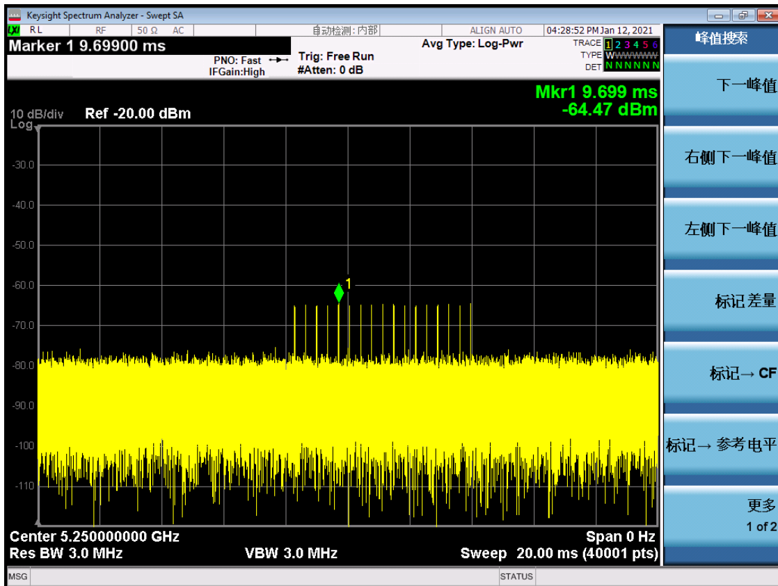
Radarsignal 3
