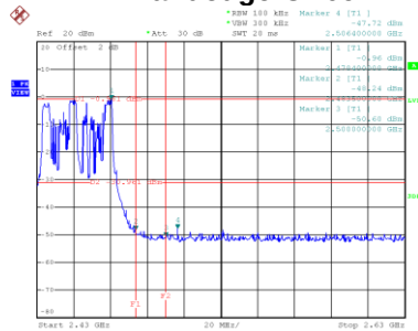
Bandedge-CH09
