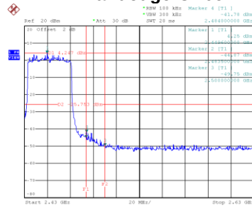
Bandedge-CH09
