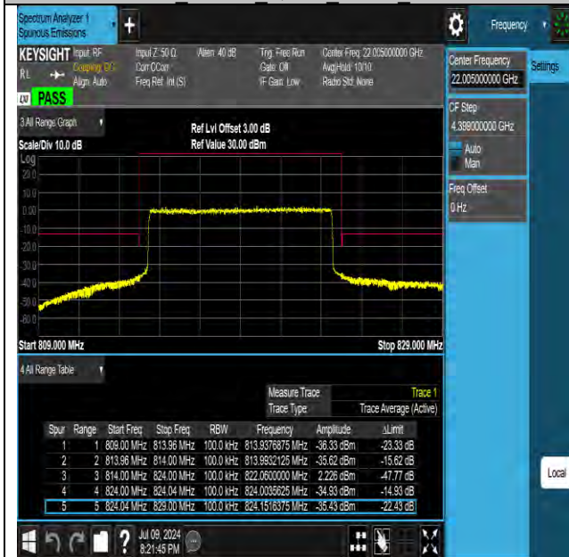
Band26 10MHz QPSK 26740 50RB#0
