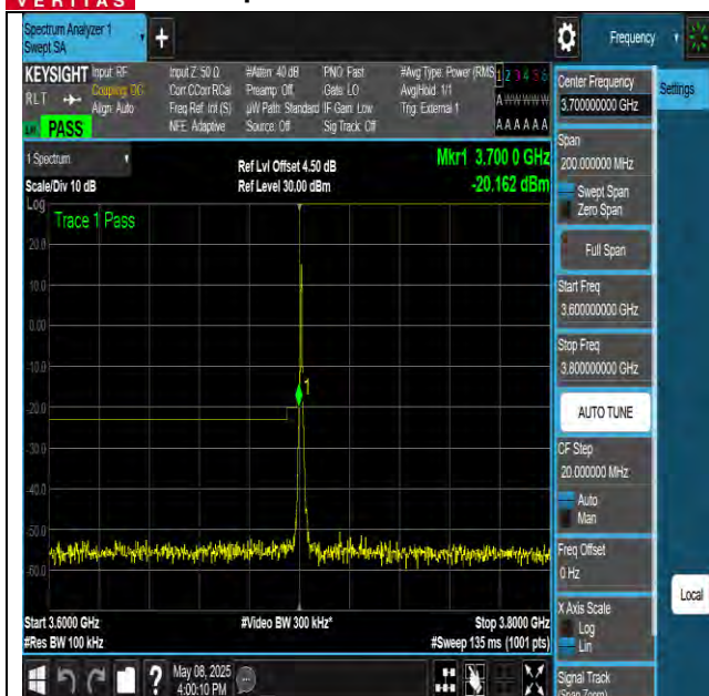
NTNV-N77-3700-3980-PC3-30-15-L-DFT-QPSK- Edge 1RB Left-Ant1-PASS
