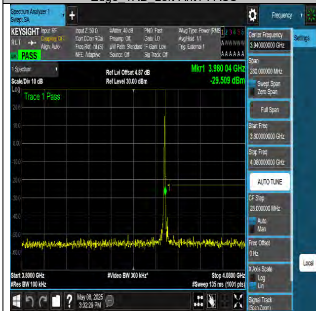
NTNV-N77-3700-3980-PC3-30-20-H-DFT-QPSK- Edge 1RB Right-Ant1-PASS
