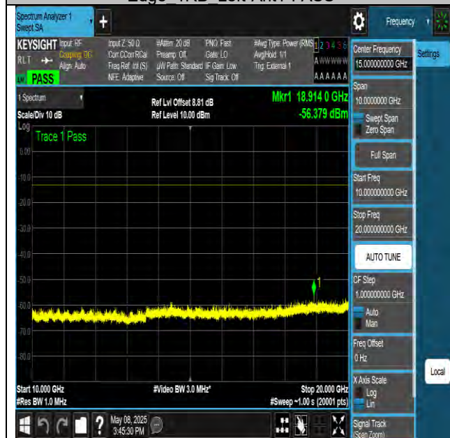
NTNV-N77-3700-3980-PC3-30-15-H-DFT-QPSK- Edge 1RB Left-Ant1-PASS
