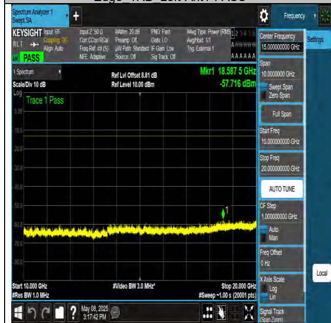
NTNV-N77-3700-3980-PC3-30-15-M-DFT-QPSK- Edge 1RB Left-Ant1-PASS
