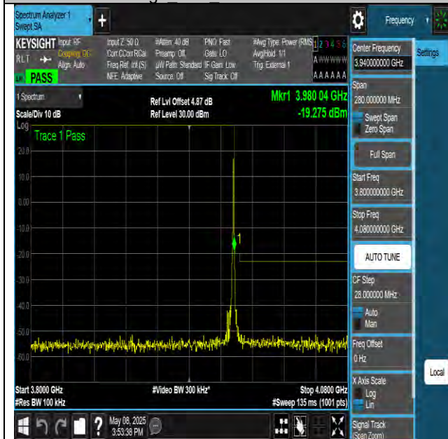
NTNV-N77-3700-3980-PC3-30-15-H-DFT-QPSK- Edge 1RB Right-Ant1-PASS
