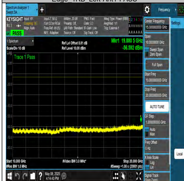
NTNV-N77-3700-3980-PC3-30-10-L-DFT-QPSK- Edge 1RB Left-Ant1-PASS
