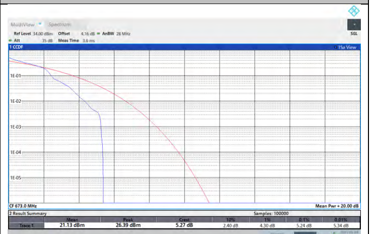
NTNV-N71-PC3-15-20-L-DFT-QPSK-Edge_1RB_Left-PASS
