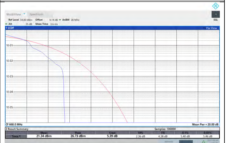
NTNV-N71-PC3-15-10-L-DFT-QPSK-Edge_1RB_Left-PASS
