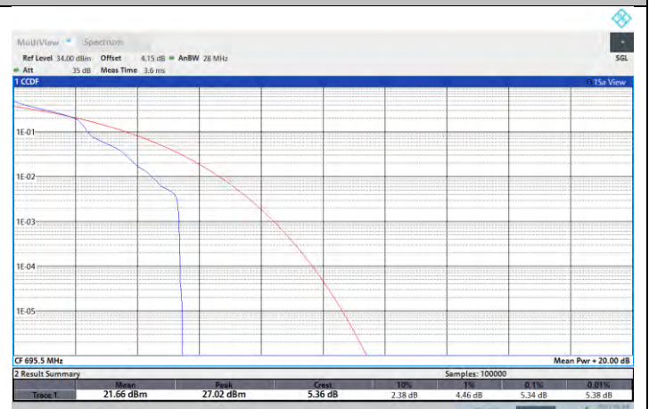
NTNV-N71-PC3-15-5-H-DFT-QPSK-Edge_1RB_Left-PASS
