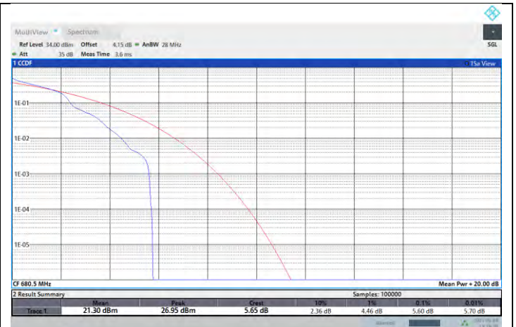
NTNV-N71-PC3-15-15-M-DFT-QPSK-Edge_1RB_Left-PASS
