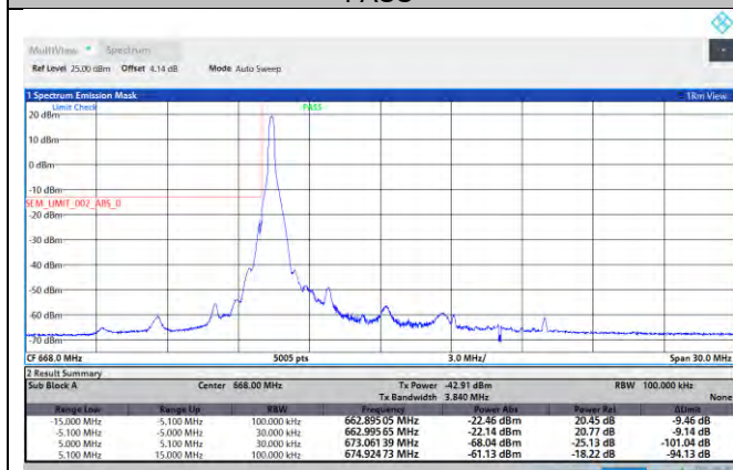
NTNV-N71-PC3-15-10-L-DFT-QPSK-Edge_1RB_Left-Ant1-PASS
