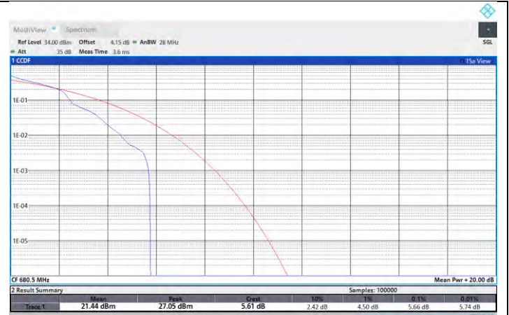
NTNV-N71-PC3-15-5-M-DFT-QPSK-Edge_1RB_Left-PASS
