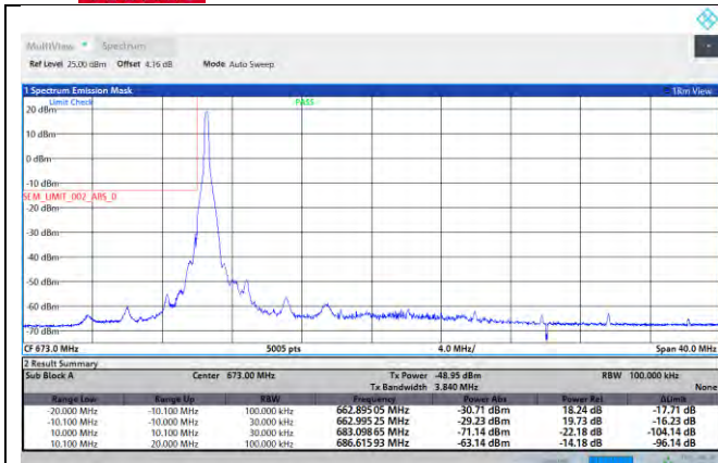
NTNV-N71-PC3-15-20-L-DFT-QPSK-Edge_1RB_Left-Ant1-PASS
