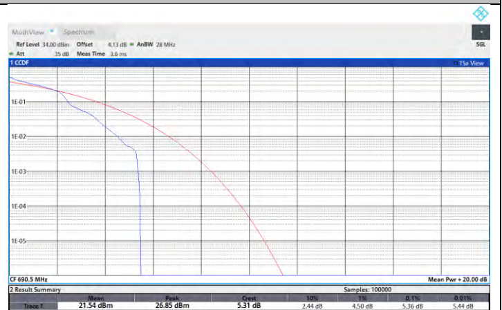
NTNV-N71-PC3-15-15-H-DFT-QPSK-Edge_1RB_Left-PASS
