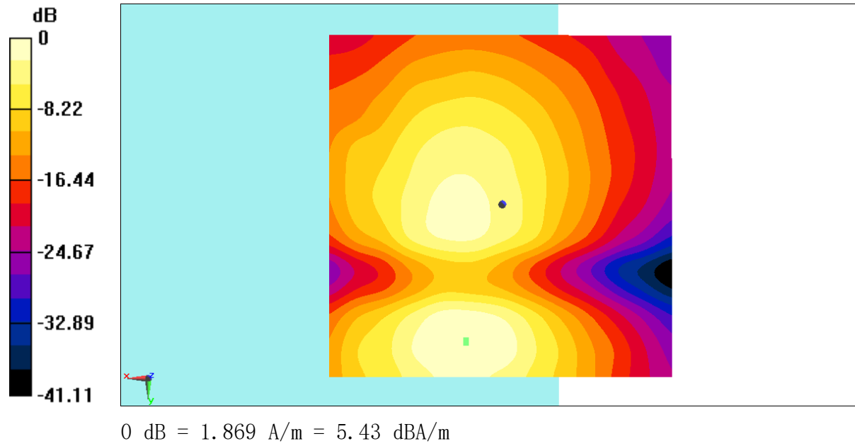
Fig B.3 T-Coil WCDMA 850
