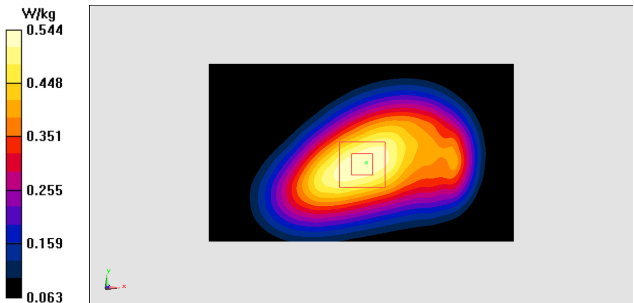
Fig.7 WCDMA 850
