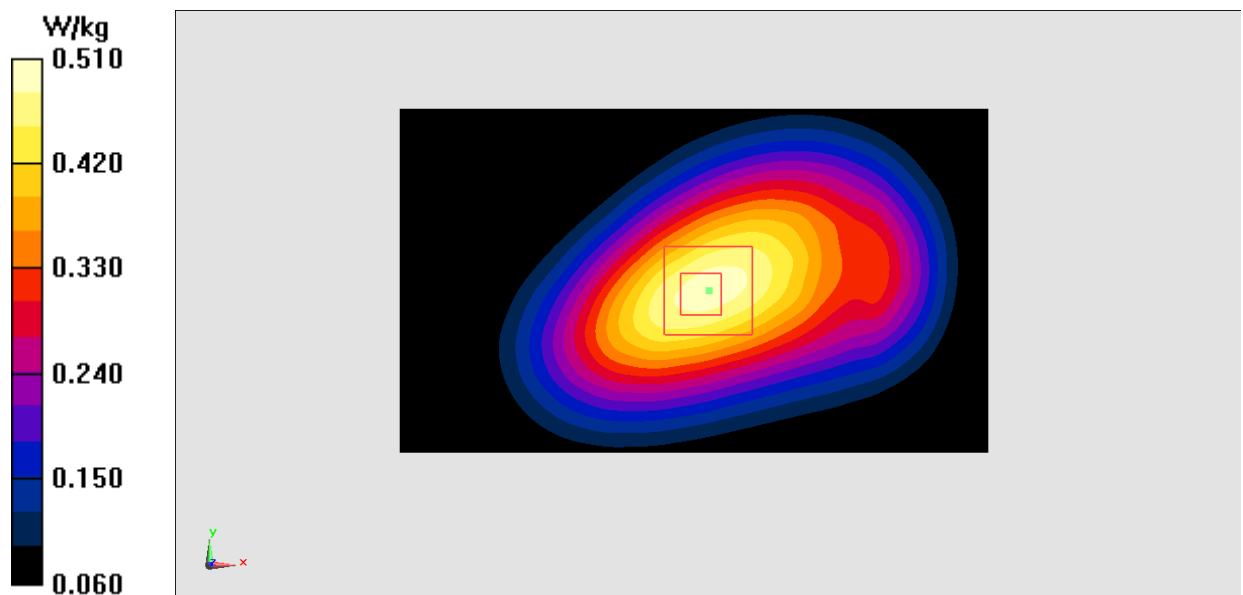
Fig.6 WCDMA 850
