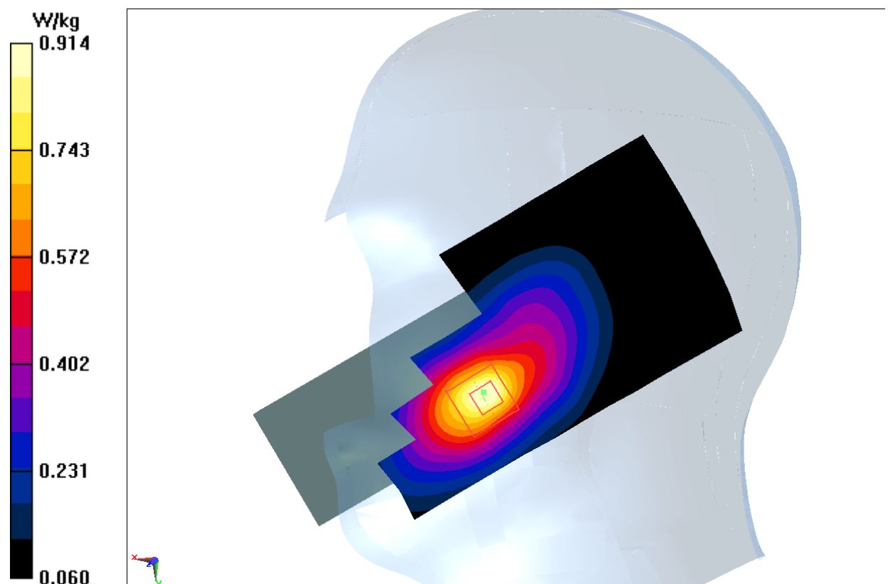
Fig.5 WCDMA 850
