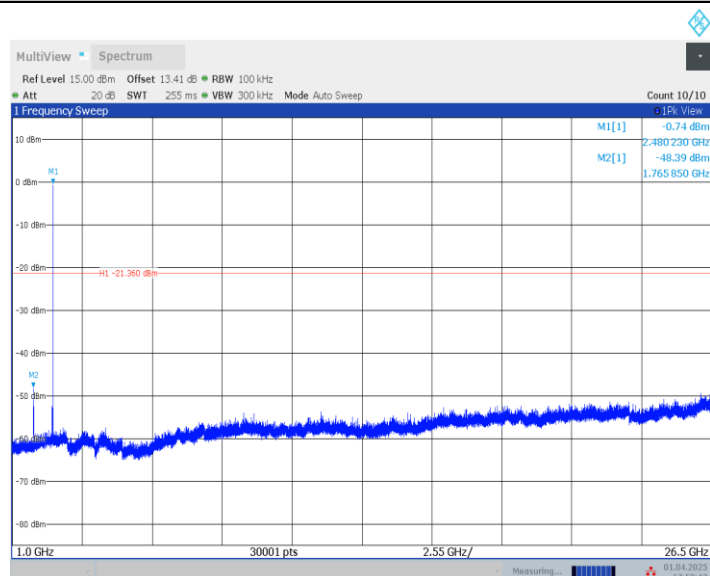
BLE_1M_Ant1_2480_1000~26500
