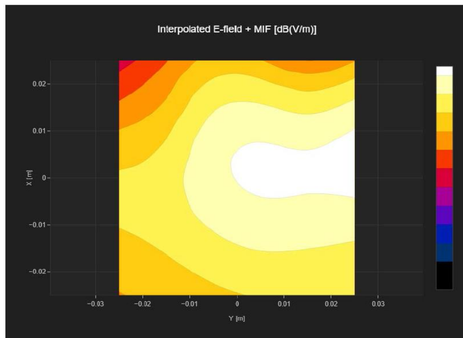
Fig B.3 NR n77 ANT2
