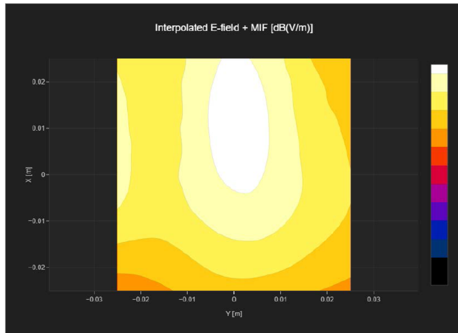
Fig B.4 NR n77 ANT6
