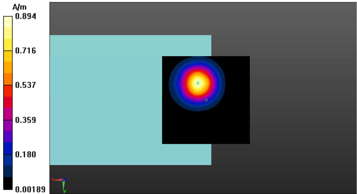
Fig A.1 T-Coil WCDMA Band 2-Z
