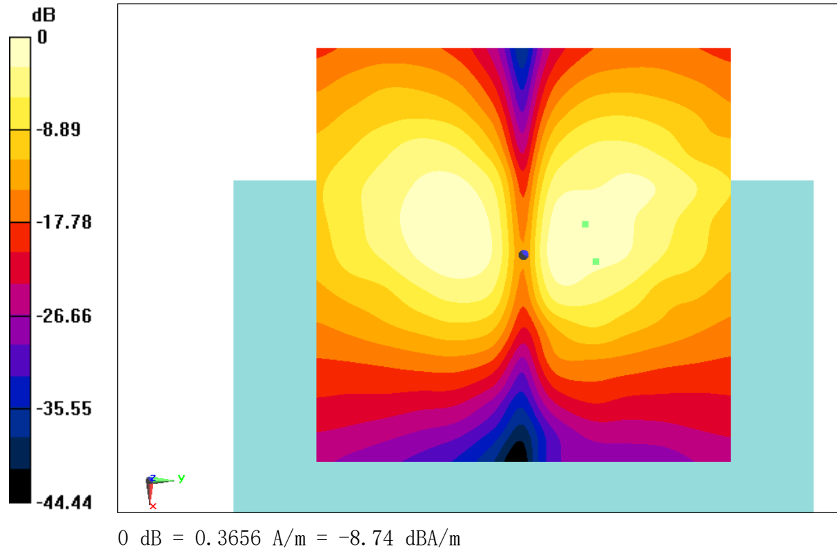
Fig B.3 T-Coil WCDMA 850
