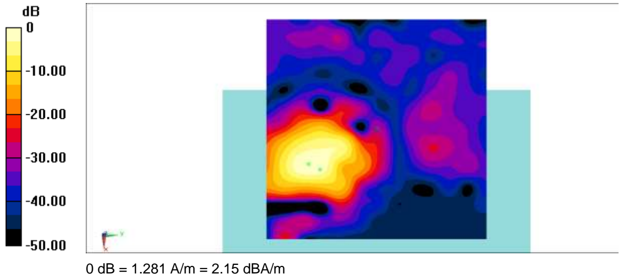
Fig B.6 T-Coil EDGE 850
