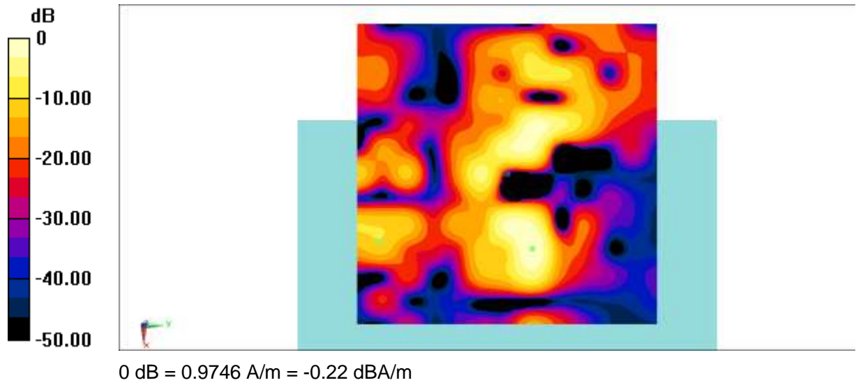
Fig B.5 T-Coil EDGE 850
