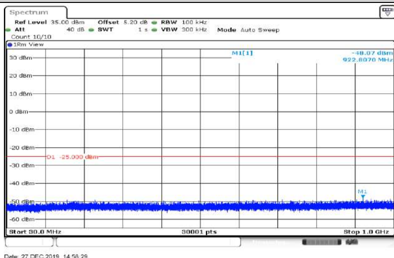
Band7-20MHz-QPSK-20850-1RB#0-Range2:1000~30000MHz
