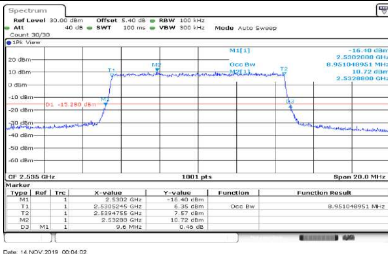
Band7-10MHz-QPSK-21400-50RB#0-8.951
