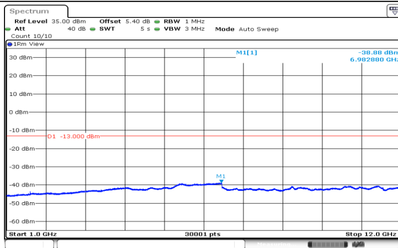
Band5-10MHz-QPSK-20450-1RB#0-Range2:1000~12000MHz
