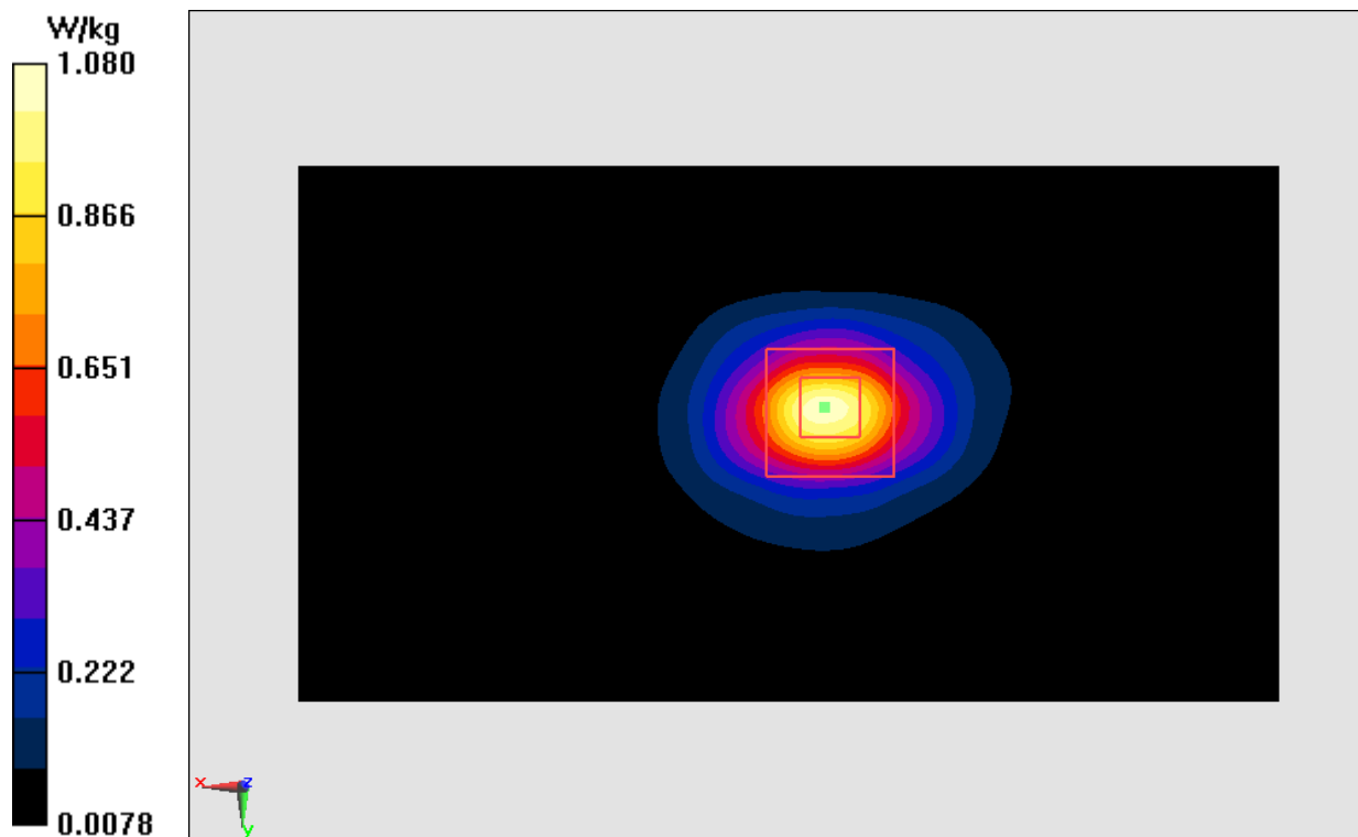
Fig.18 LTE Band7
