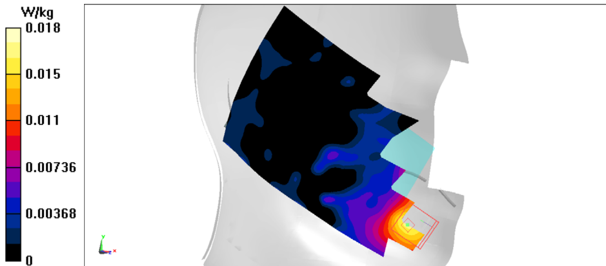
Fig.17 LTE Band7
