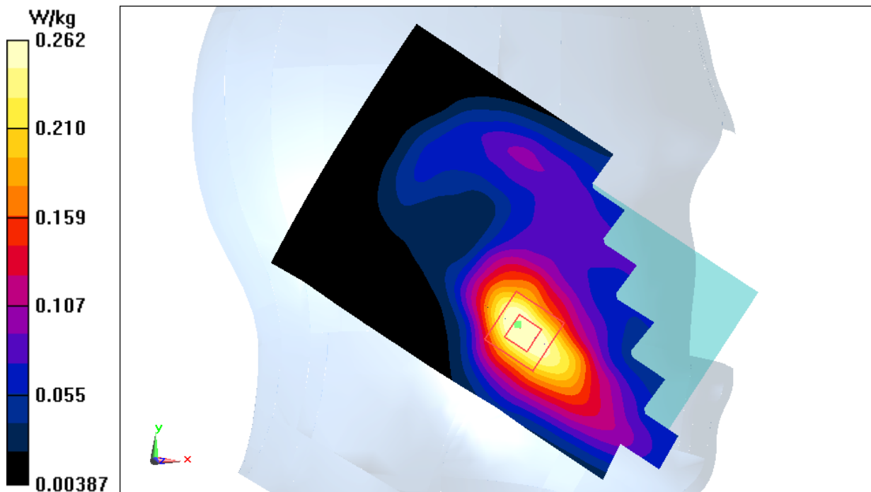
Fig.13 LTE Band4
