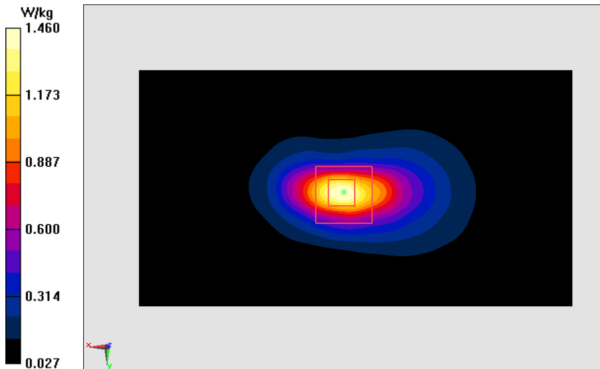
Fig.14 LTE Band4
