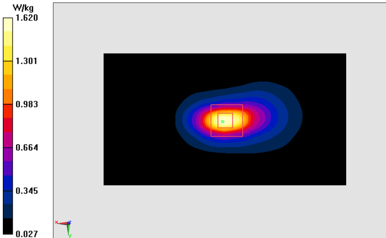
Fig.10 WCDMA1900
