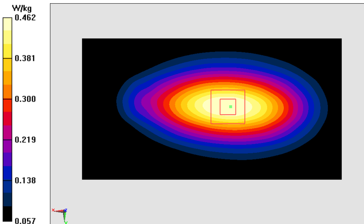
Fig.16 LTE Band5
