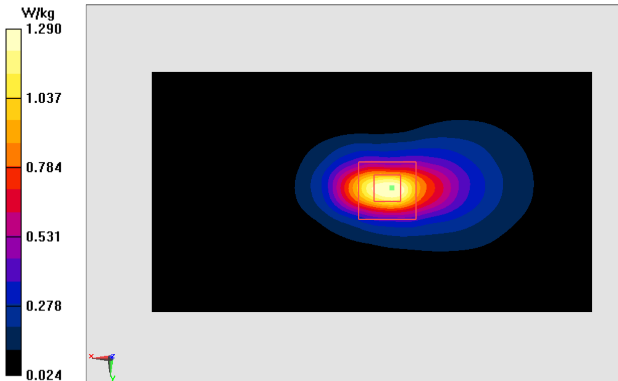
Fig.12 LTE Band2
