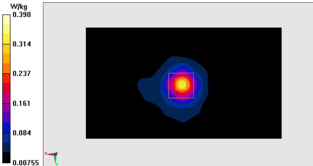
Fig.24 5GHz
