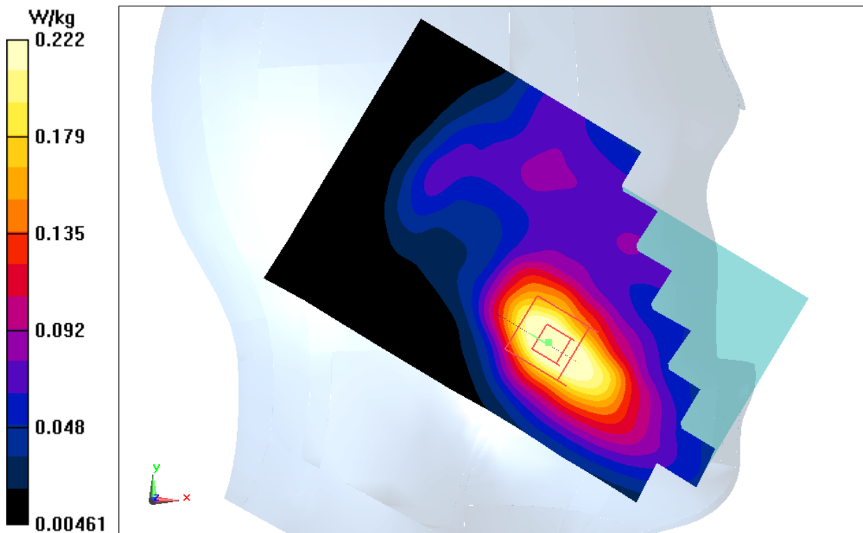
Fig.7 WCDMA1700
