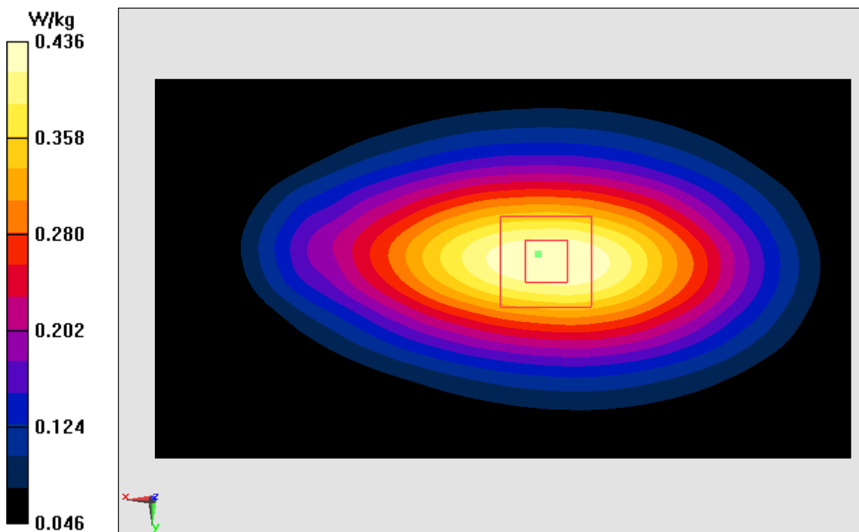
Fig.6 WCDMA 850
