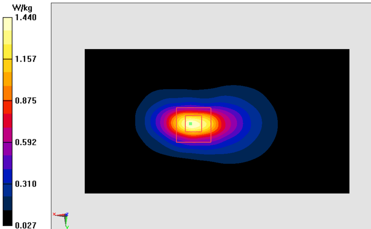
Fig.8 WCDMA1700
