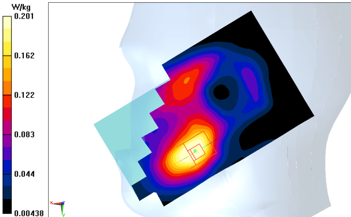
Fig.9 WCDMA1900
