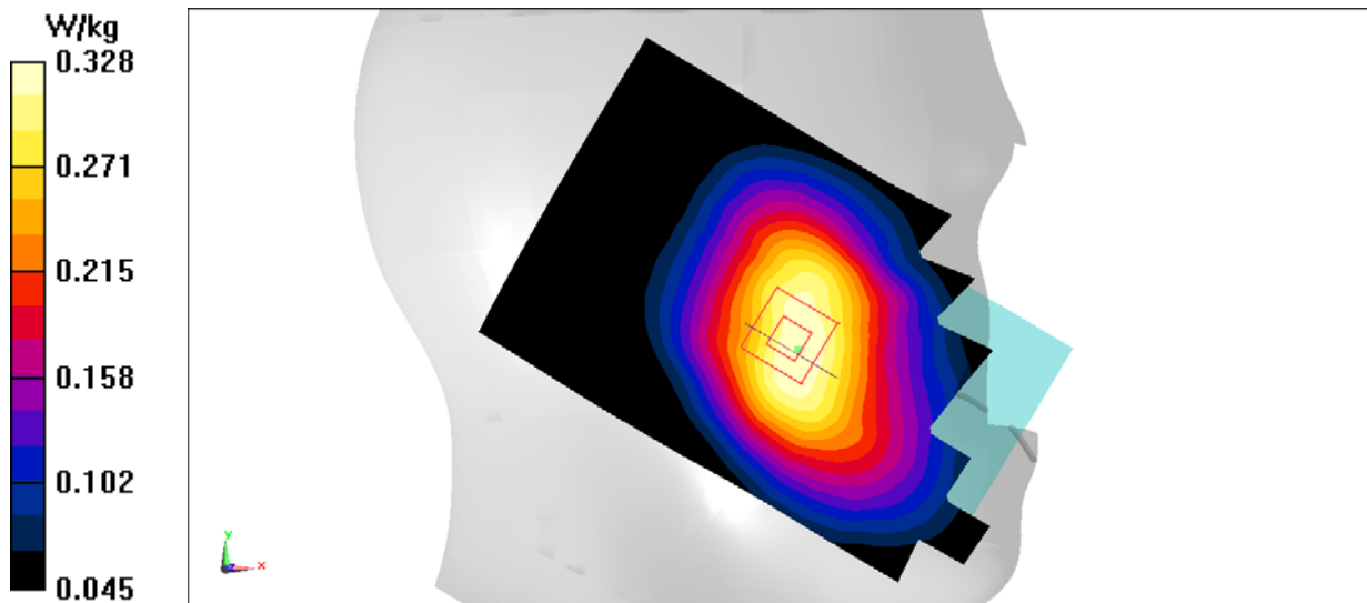
Fig.15 LTE Band5
