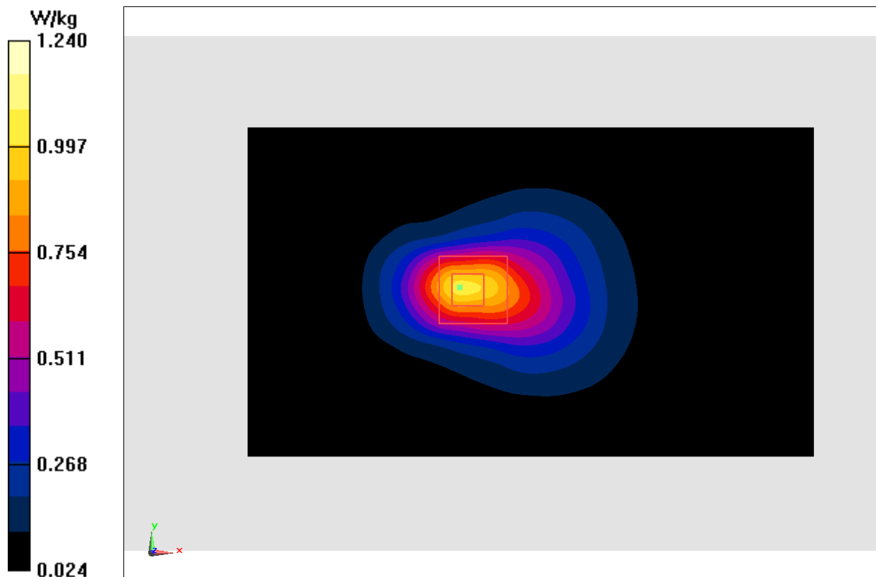
Fig.12 LTE Band4
